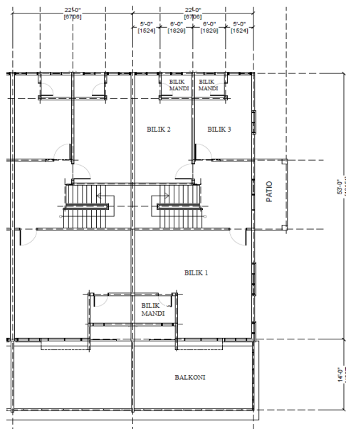
TINGKAT ATAS
