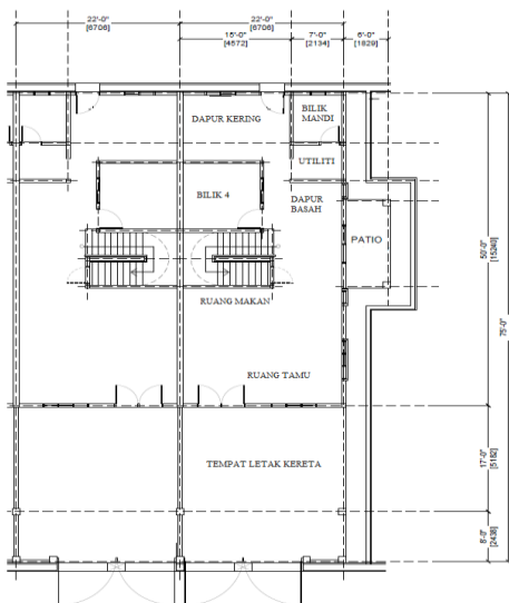
TINGKAT BAWAH
