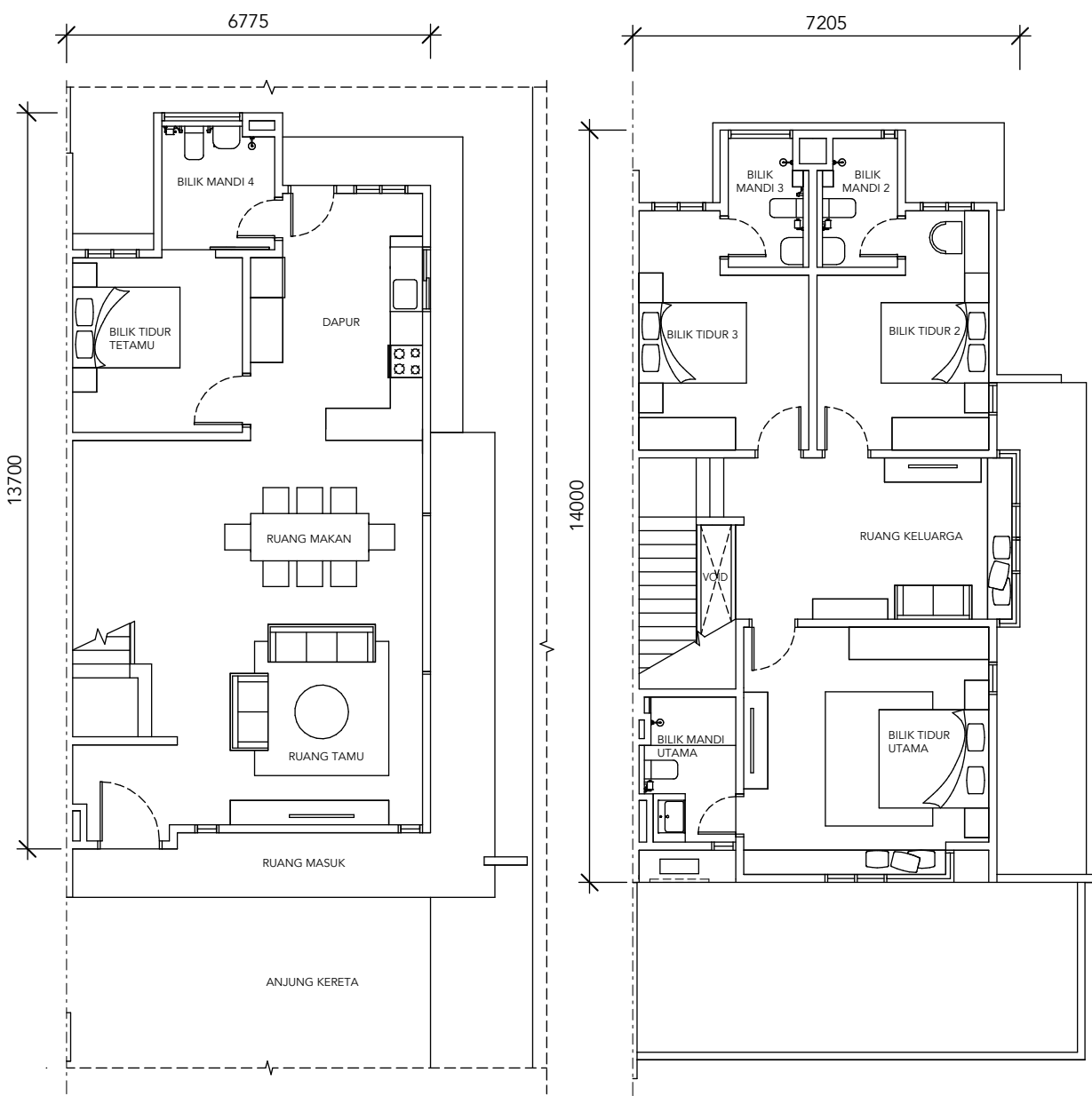
Tingkat Bawah
