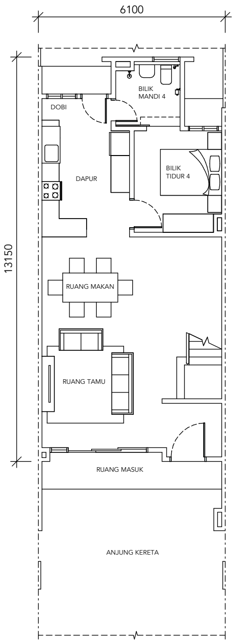
Tingkat Bawah
