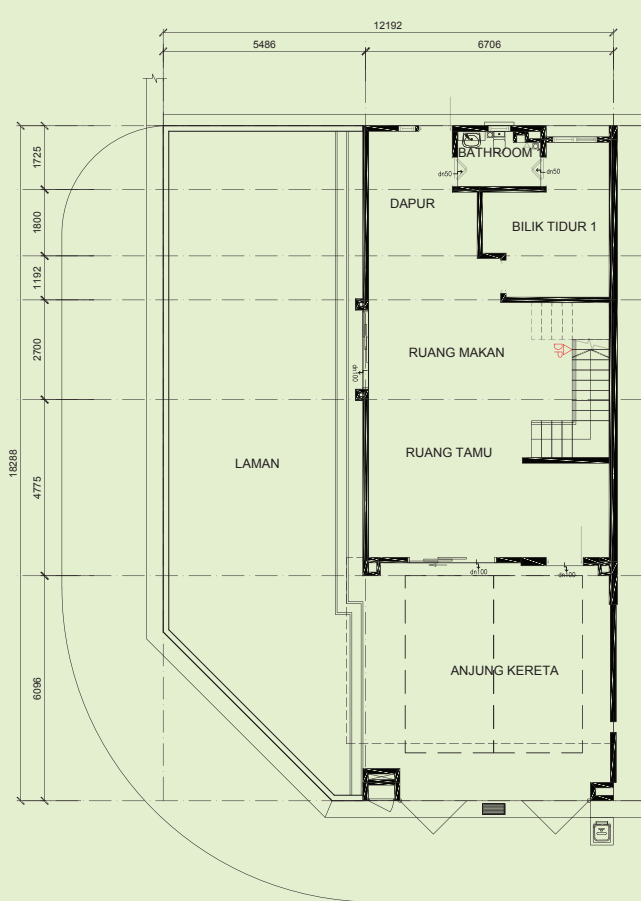
Tingkat Bawah
