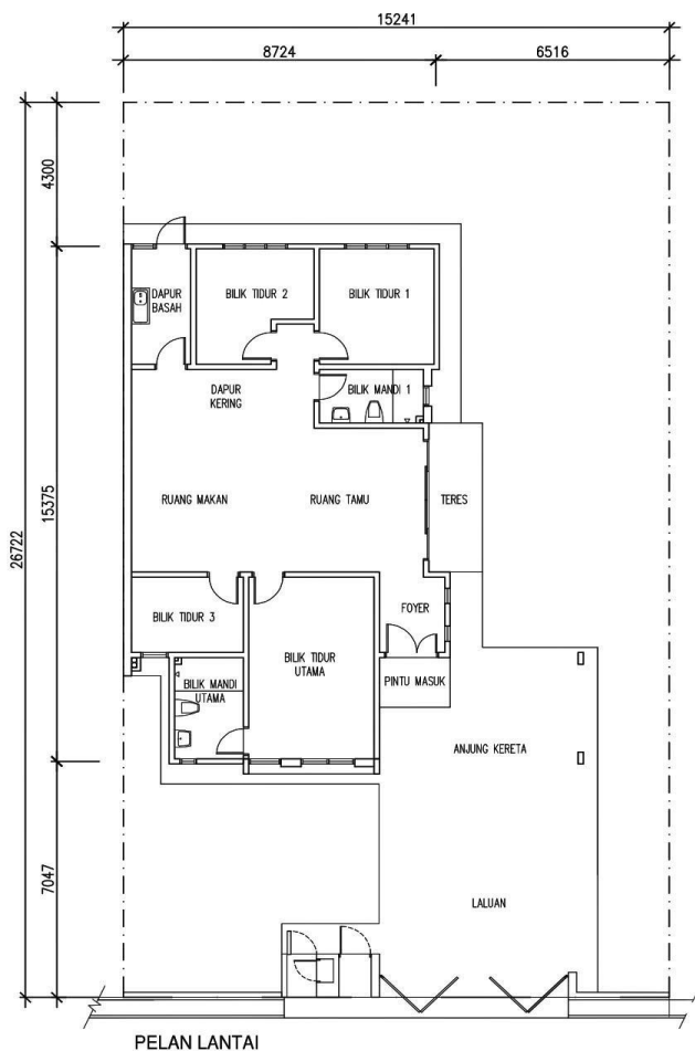
PELAN LANTAI
