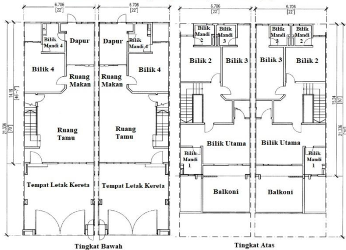
Pelan Lantai
