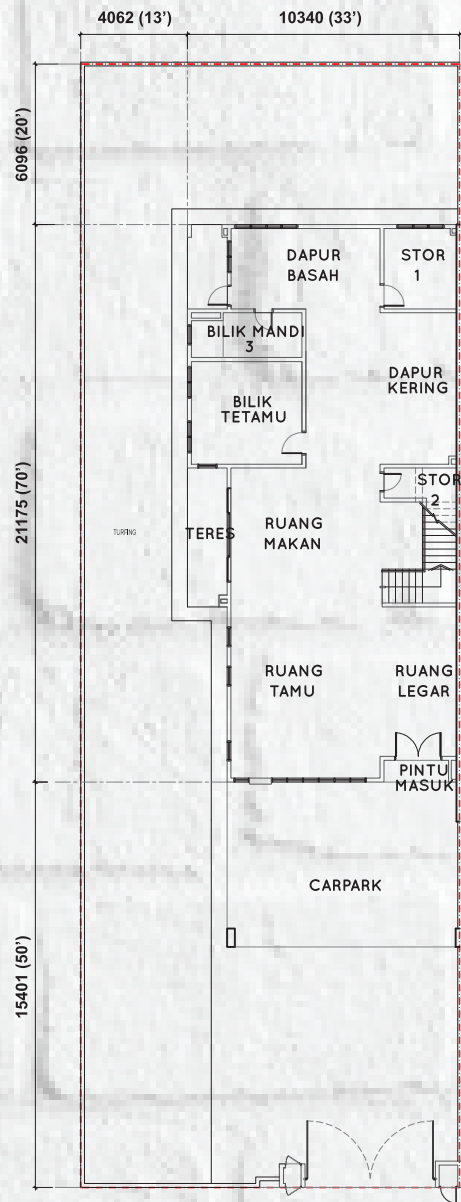
Tingkat Bawah
