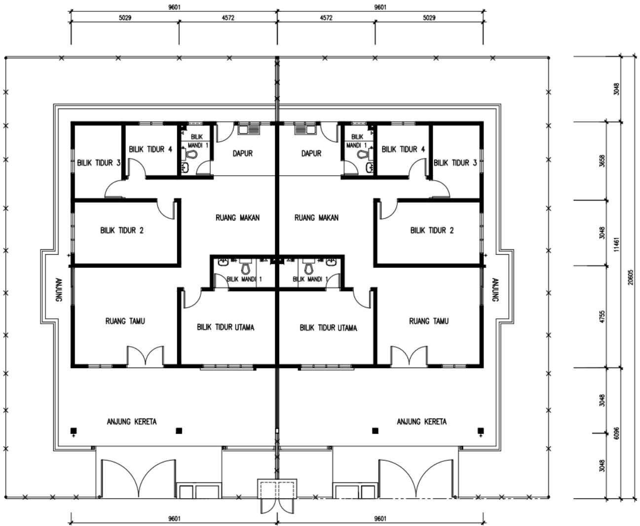
PELAN ARAS LANTAI
