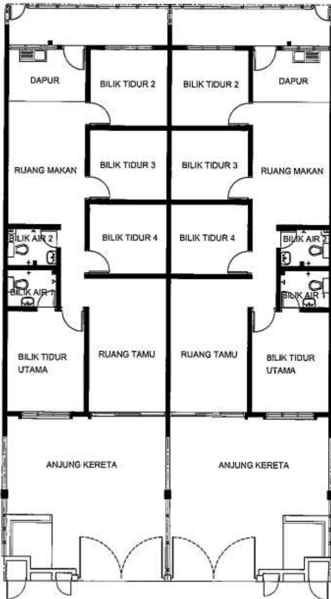
PELAN ARAS TINGKAT BAWAH
