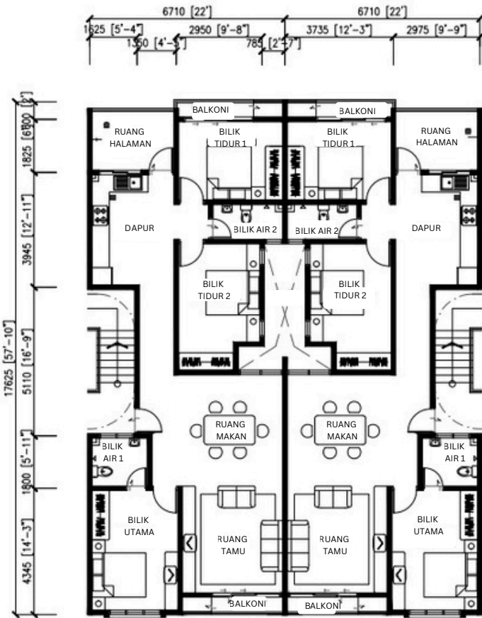
PELAN LANTAI (ARAS DUA)
