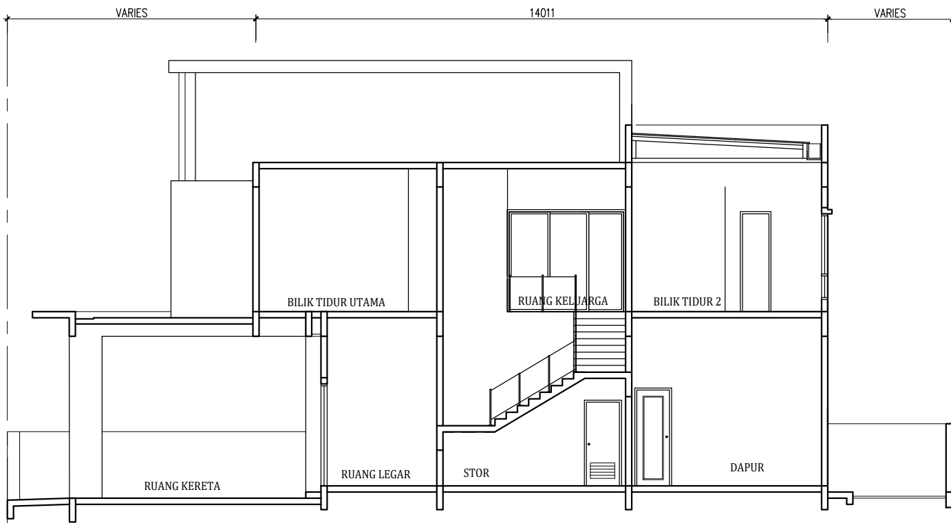
KERATAN
