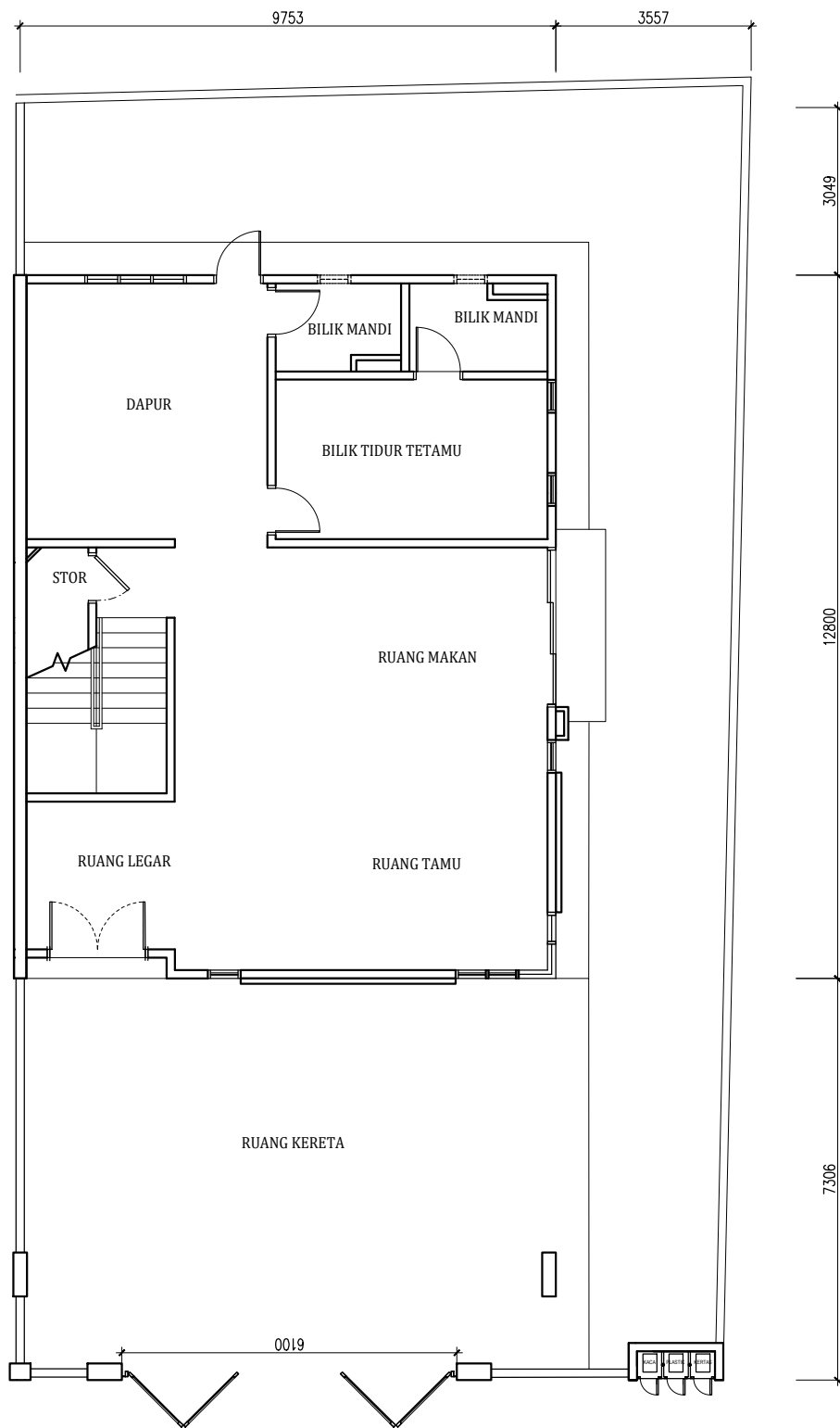
PELAN LANTAI
