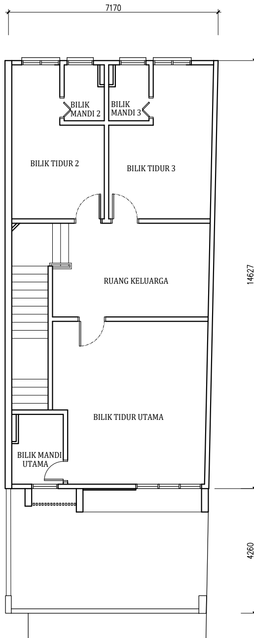
PELAN LANTAI
