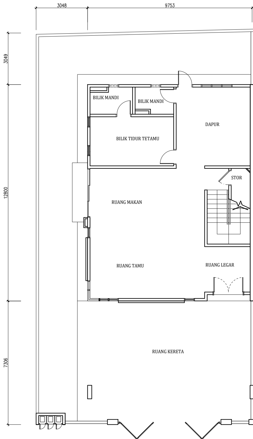
PELAN LANTAI
