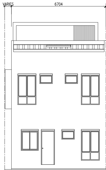
PANDANGAN BELAKANG
