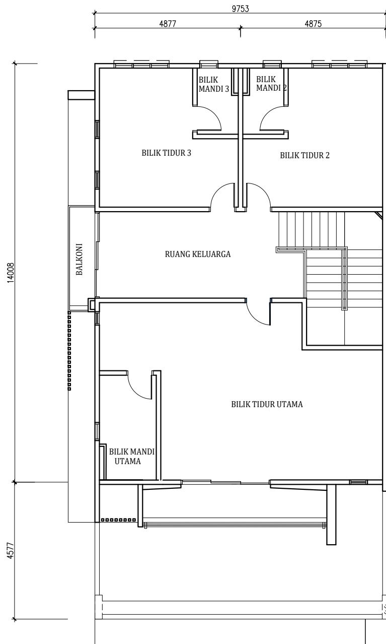
PELAN LANTAI
