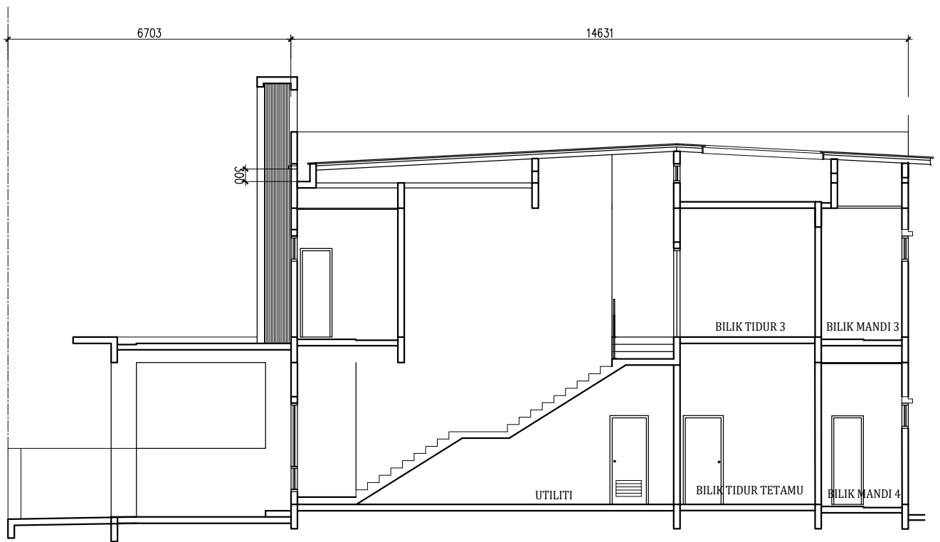
KERATAN
