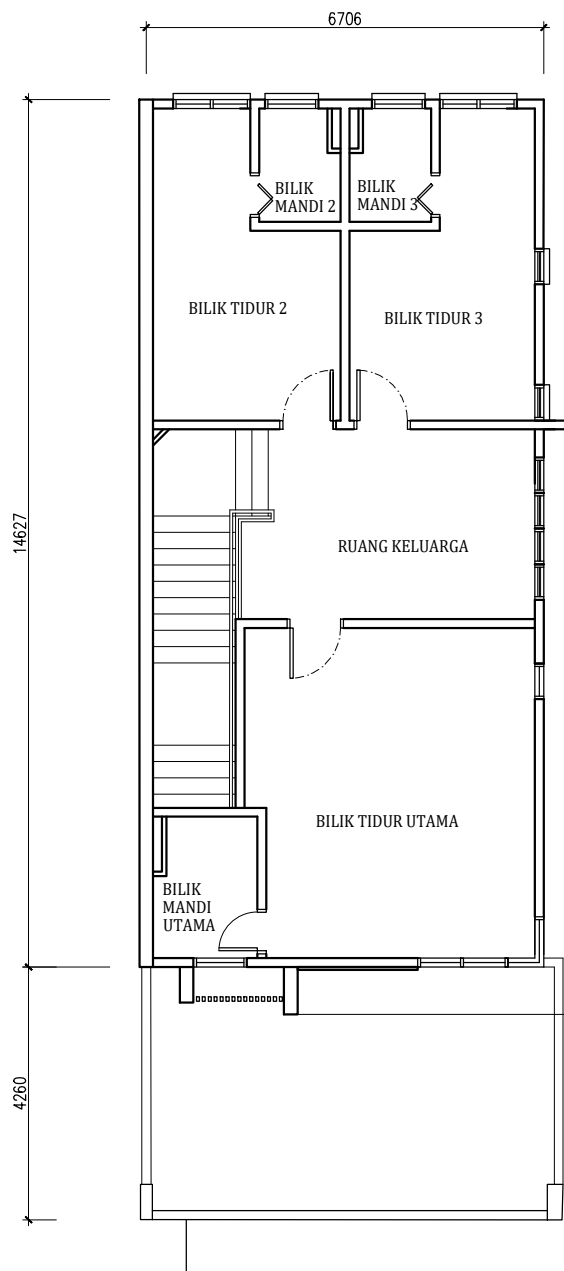
PELAN LANTAI
