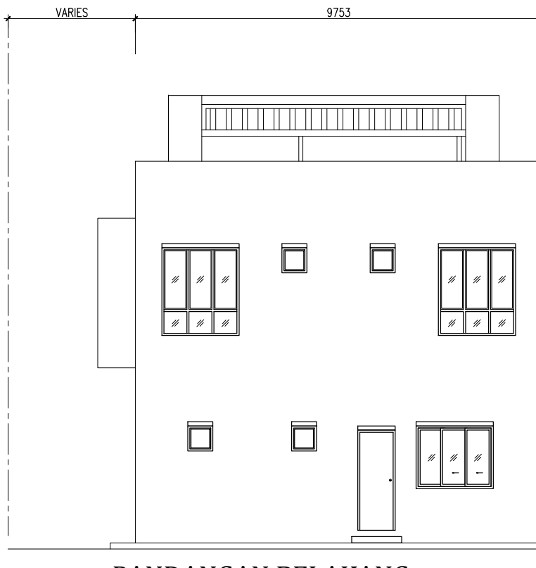
PANDANGAN BELAKANG
