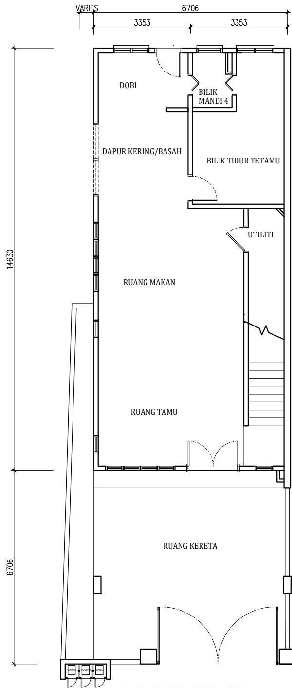
PELAN LANTAI
