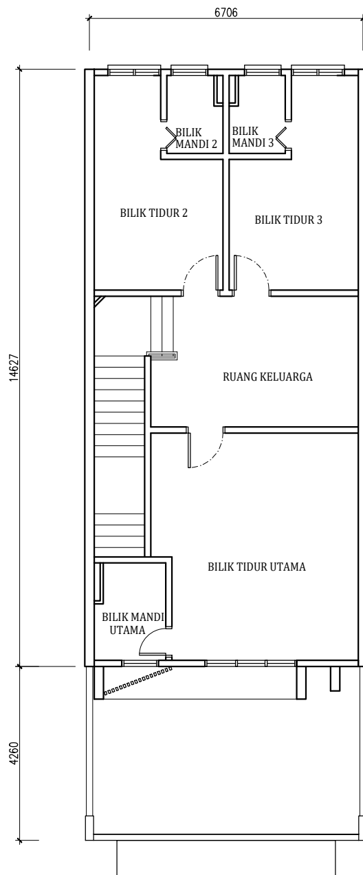
PELAN LANTAI
