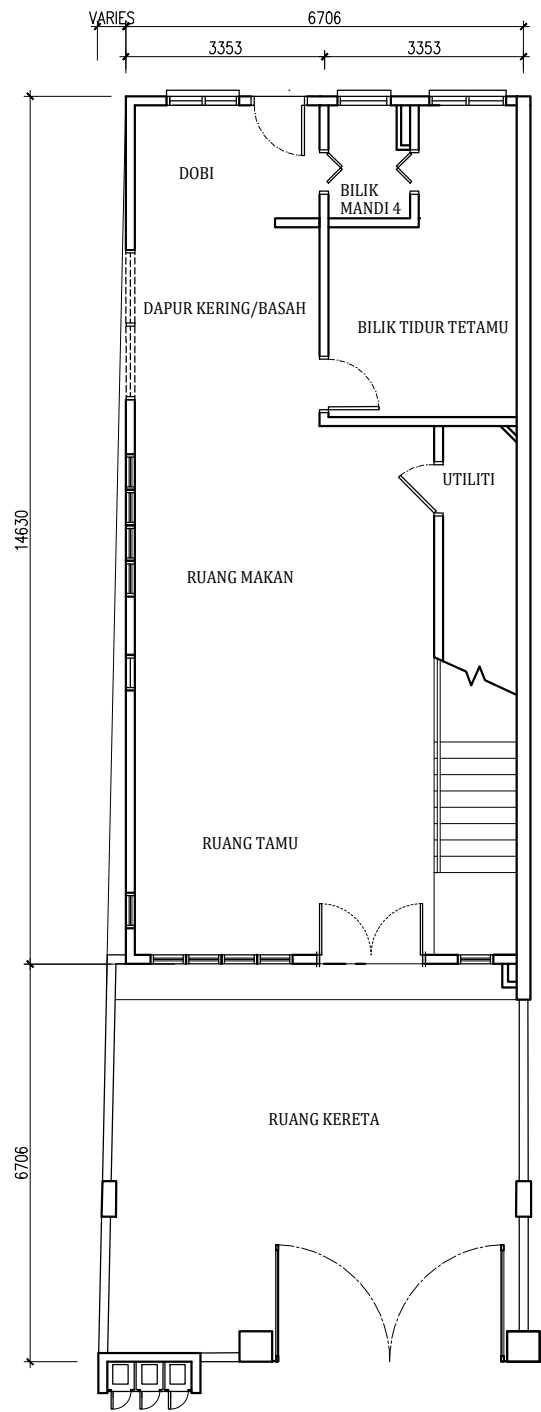
PELAN LANTAI
