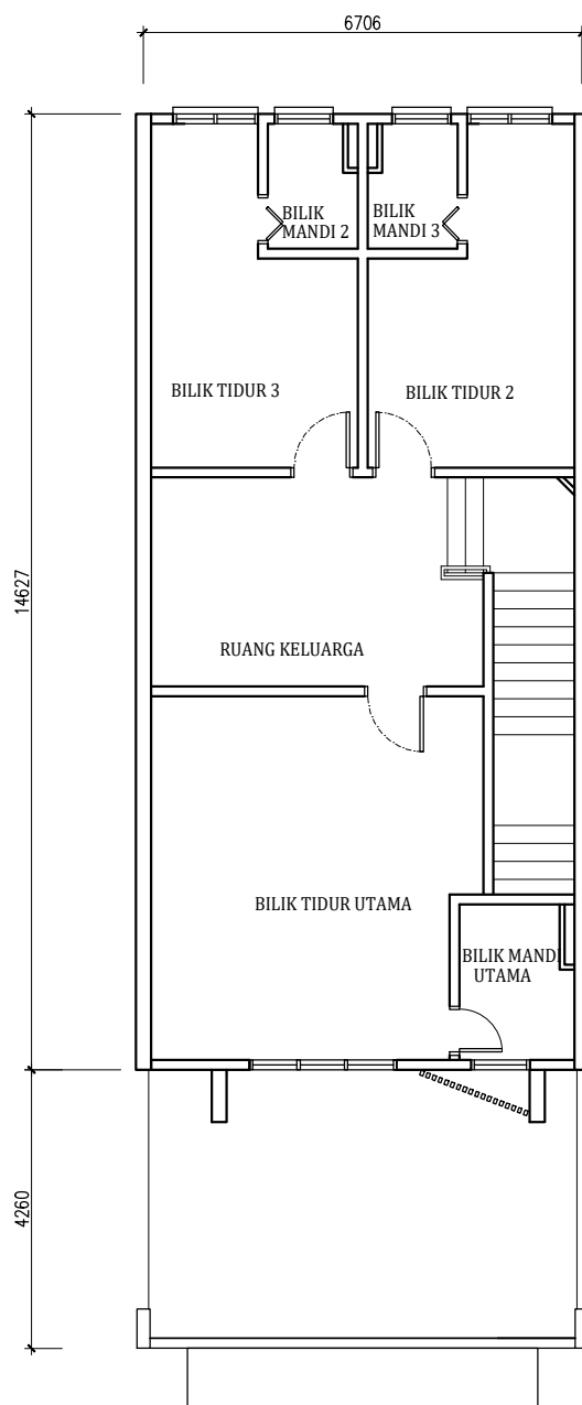
PELAN LANTAI
