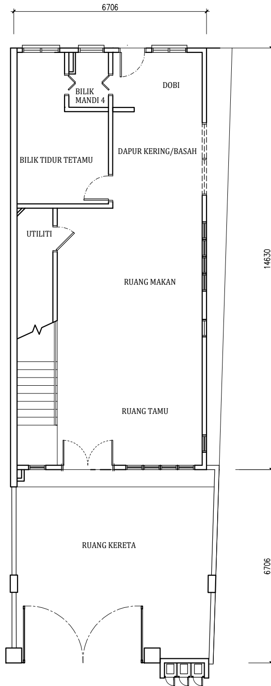
PELAN LANTAI
