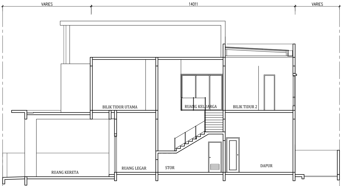
KERATAN
