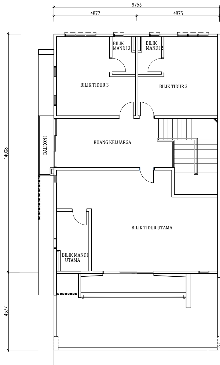
PELAN LANTAI
