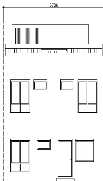
PANDANGAN BELAKANG
