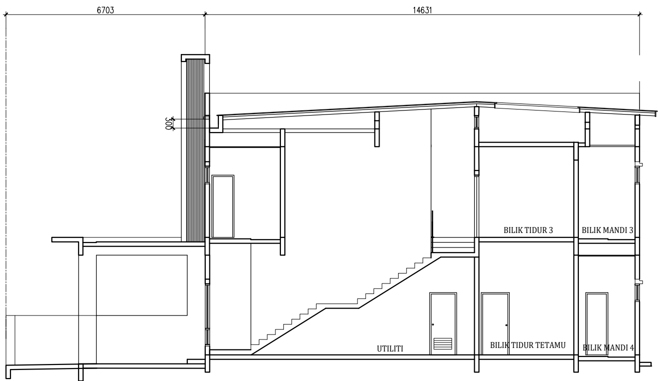
KERATAN
