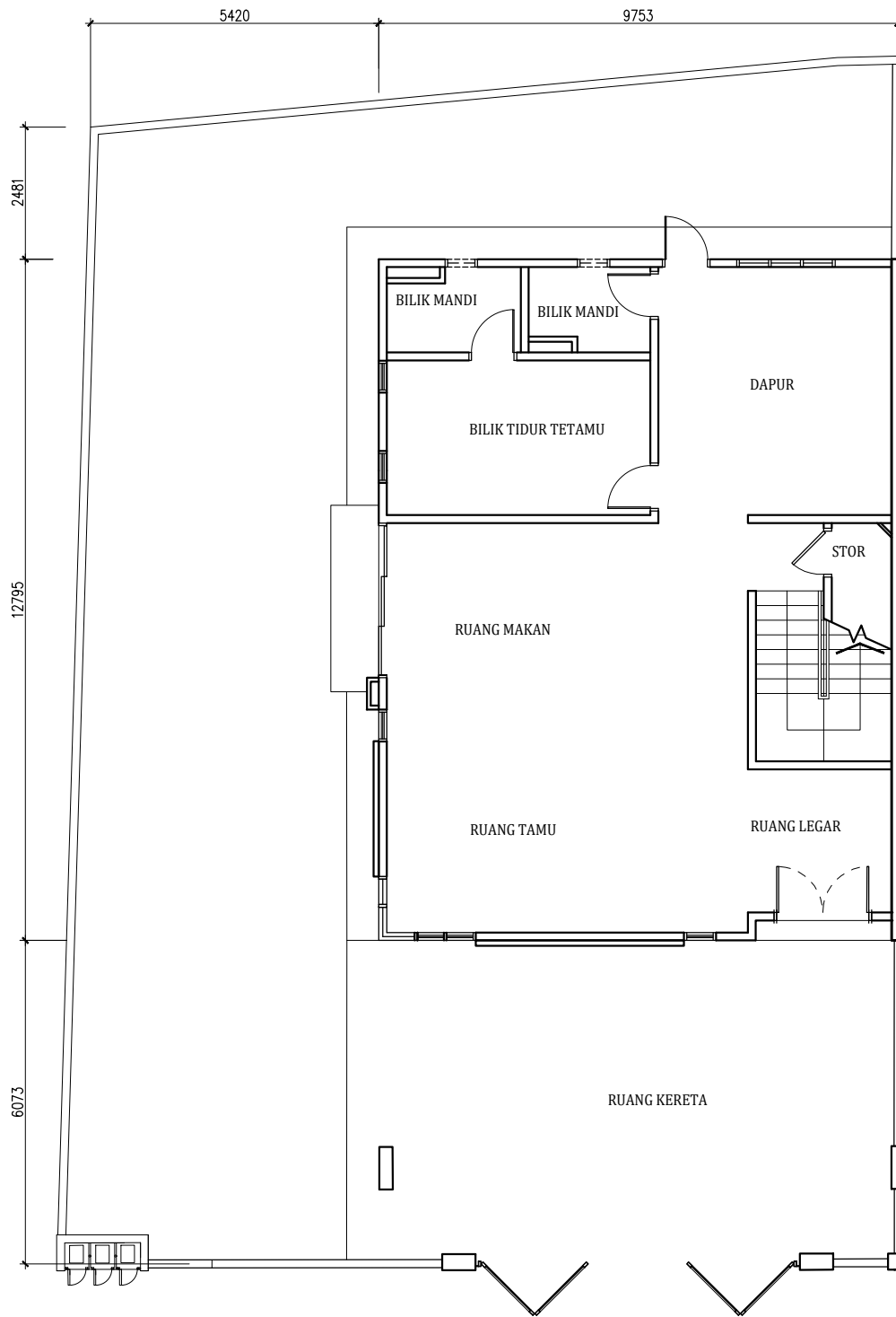
PELAN LANTAI
