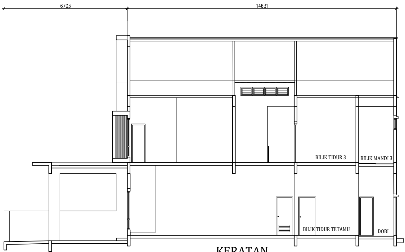
KERATAN
