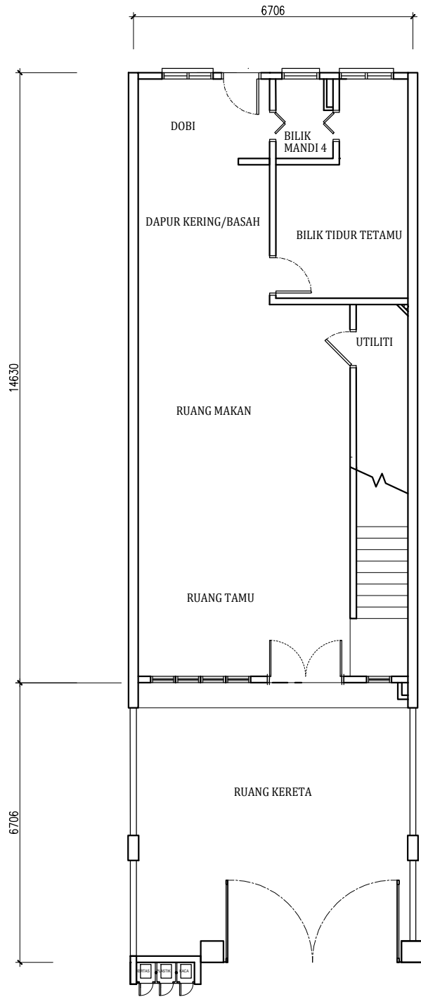
PELAN LANTAI
