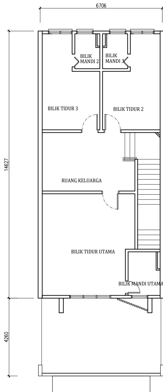
PELAN LANTAI
