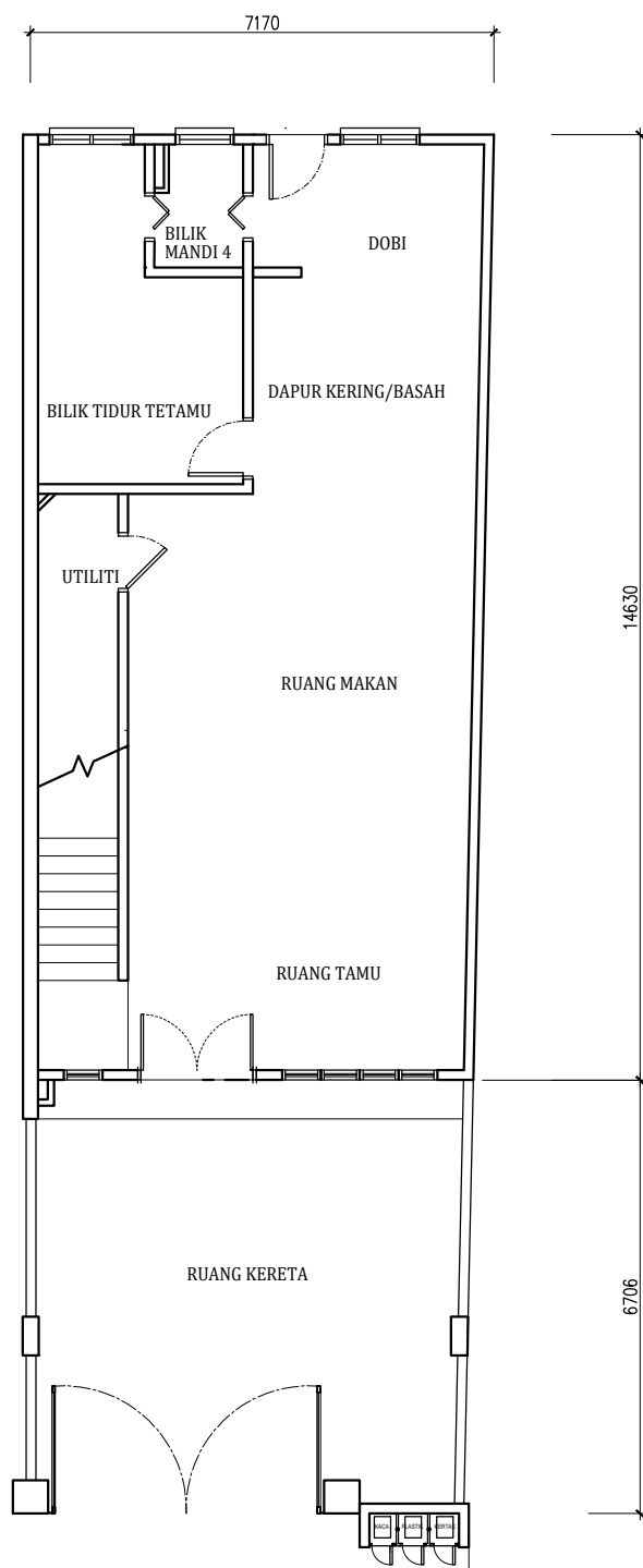
PELAN LANTAI
