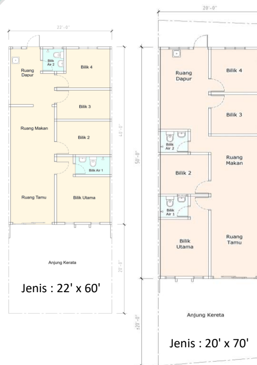
PELAN LANTAI (Lot Tengah)
