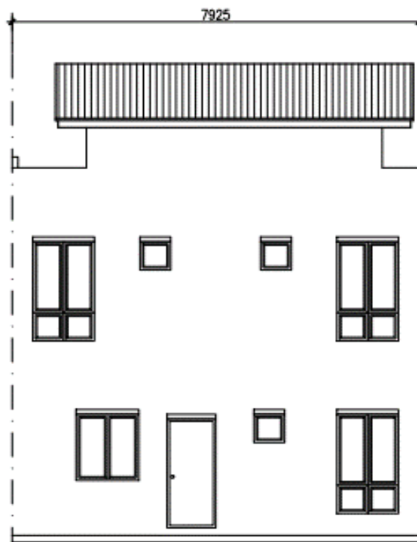
PANDANGAN BELAKANG
