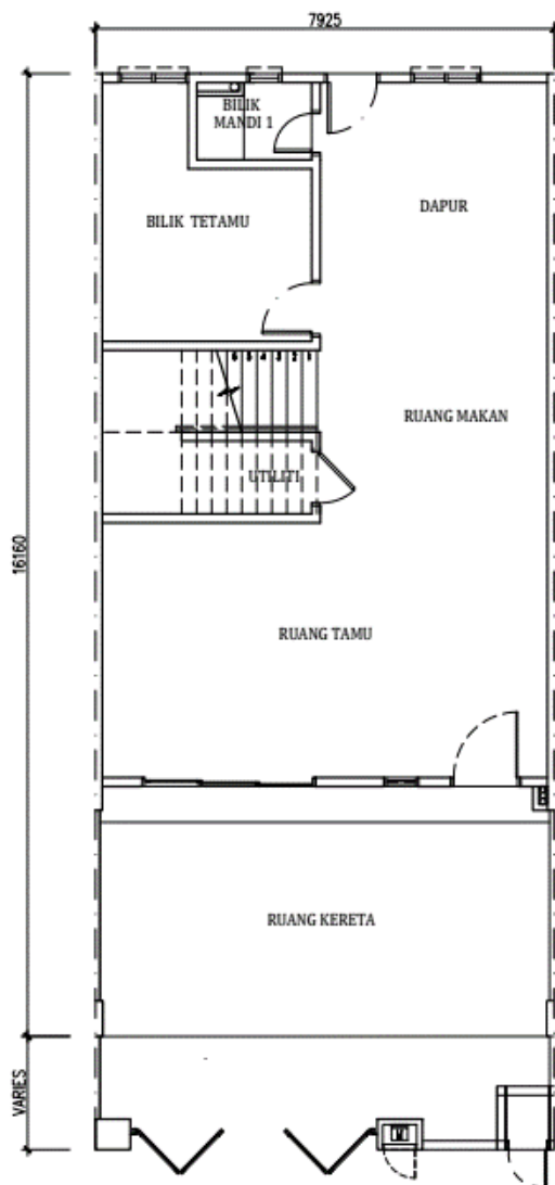
PELAN LANTAI
