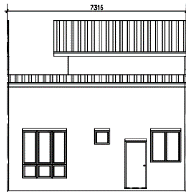
PANDANGAN BELAKANG
