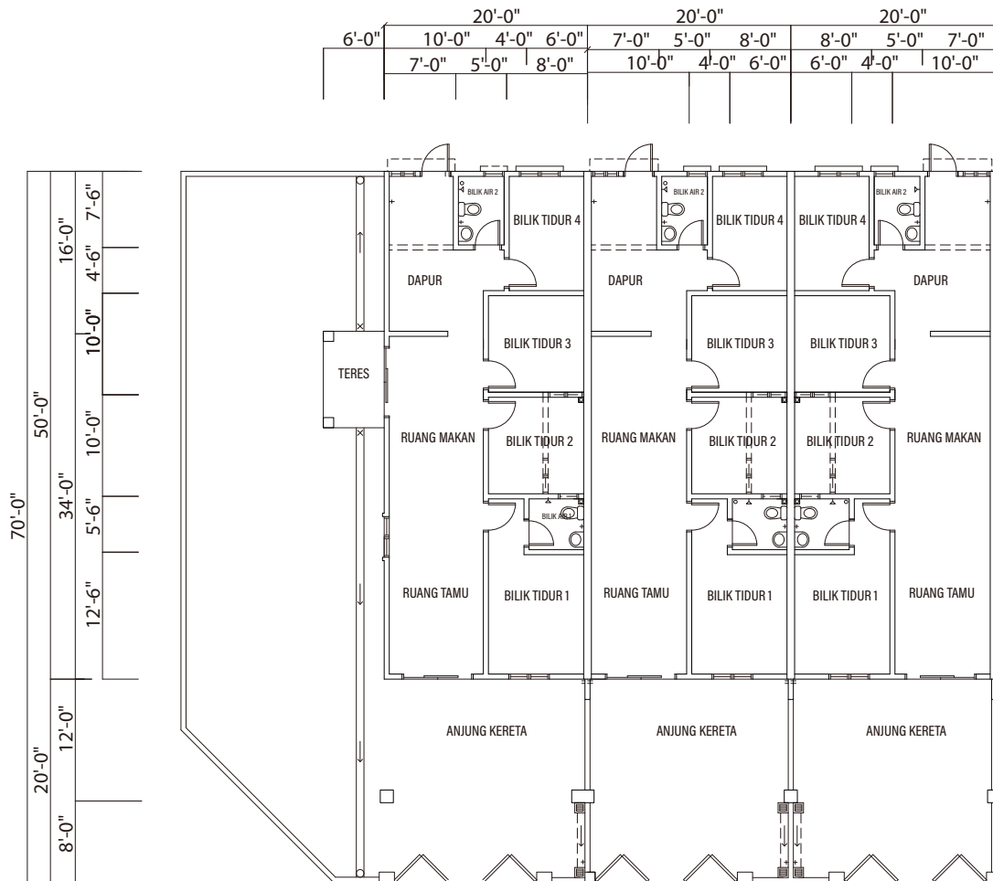
PELAN LANTAI
