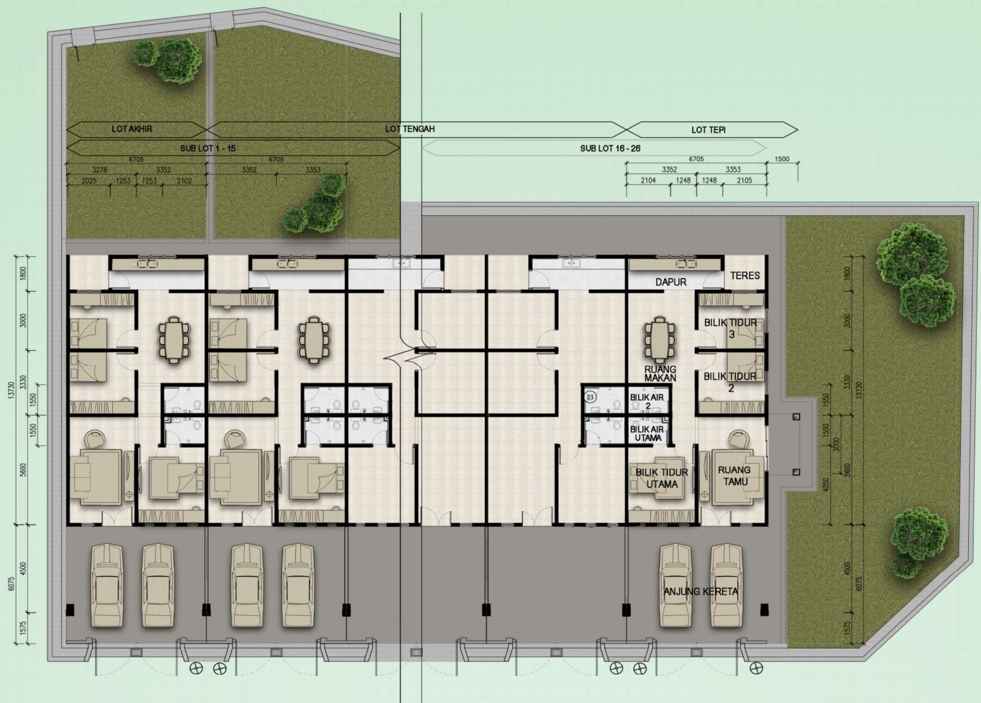
PELAN LANTAI SKALA 1 : 100
