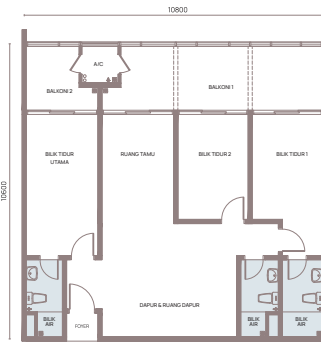
JENIS E JUMLAH KAWASAN 114.48m | 1,233kp
