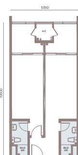
JENIS SUITE HOMES 5 JUMLAH KAWASAN 56.71m | 610kp
