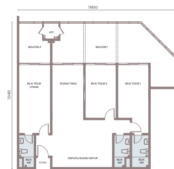
JENIS C JUMLAH KAWASAN 148.27m | 1,596kp
