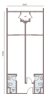
JENIS SUITE HOMES 2 JUMLAH KAWASAN 70.49m | 759kp
