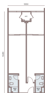
JENIS SUITE HOMES 1 JUMLAH KAWASAN 69.23m | 745kp
