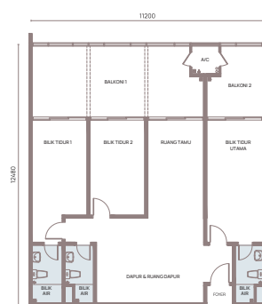
JENIS B JUMLAH KAWASAN 139.72m | 1,504kp
