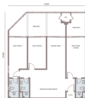
JENIS A JUMLAH KAWASAN 136.26m | 1,467kp
