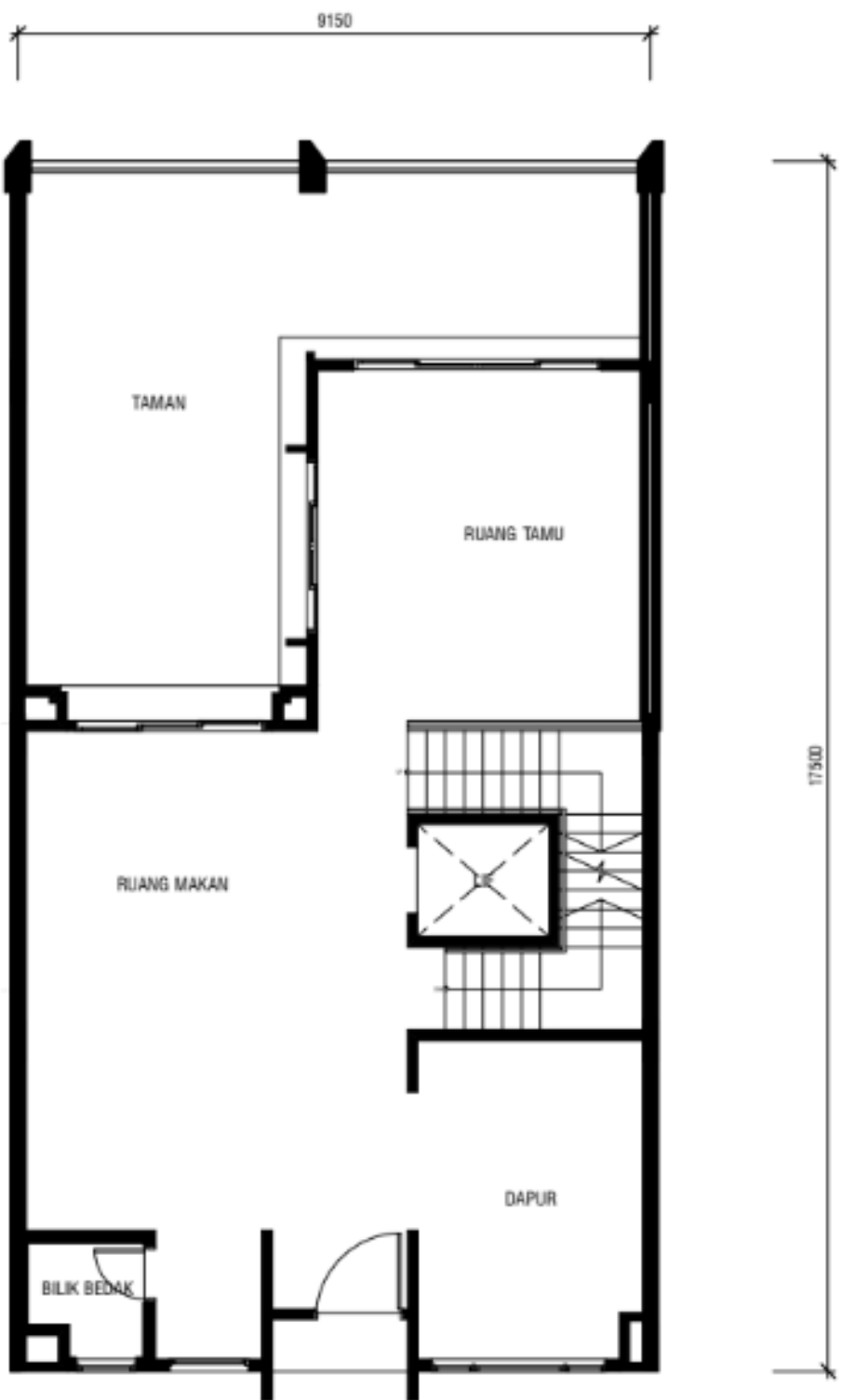
PELAN TINGKAT BAWAH
