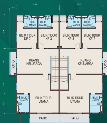
Pelan Tingkat Satu
