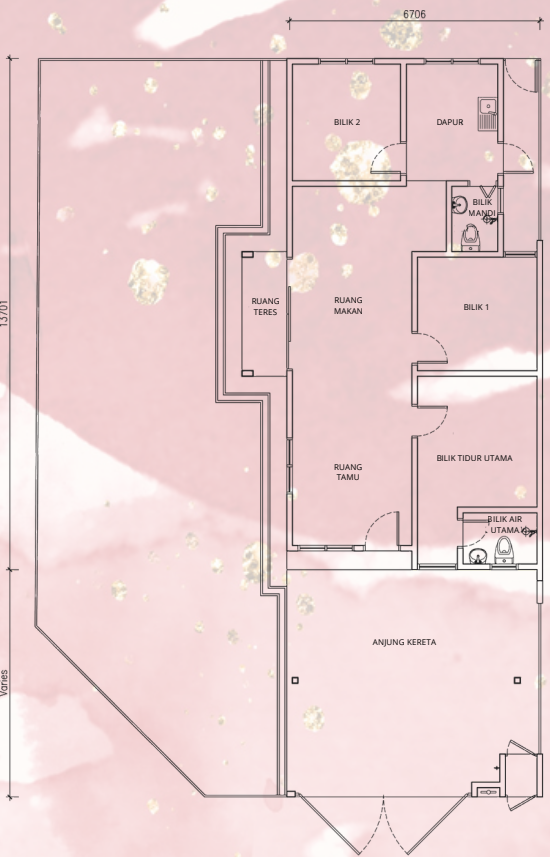
JENIS F1 1,267 k.p.s. | 3 Bilik, 2 Bilik Air
