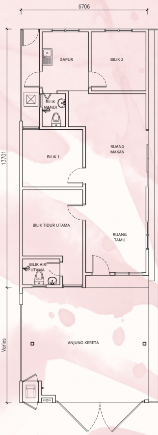
JENIS F4 1,183 k.p.s. | 3 Bilik, 2 Bilik Air
