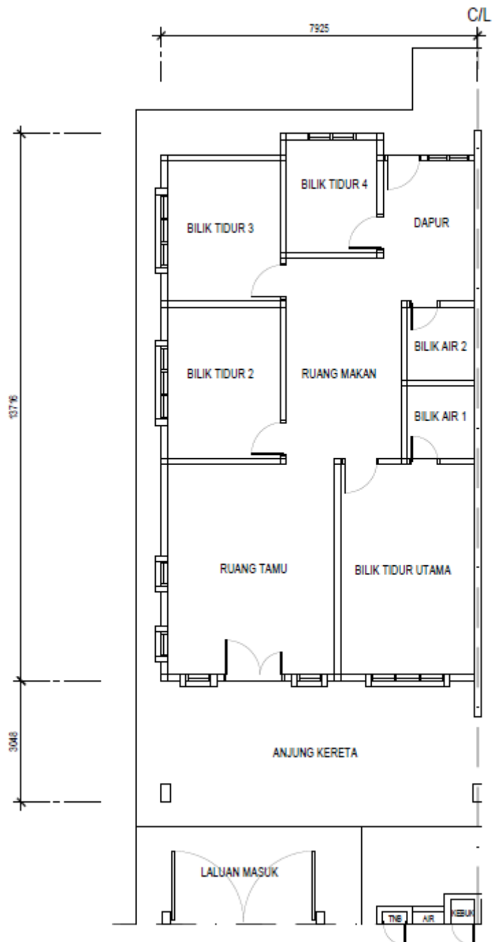
PELAN LANTAI
