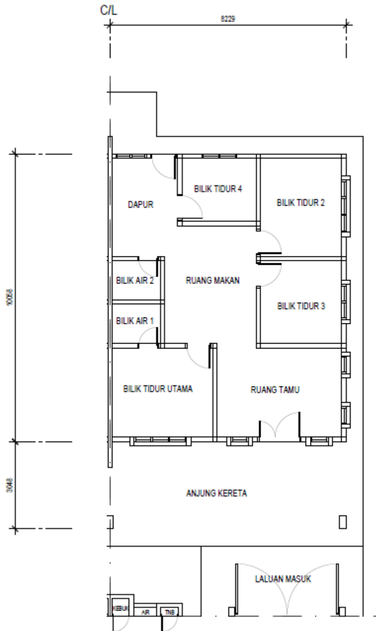
PELAN LANTAI
