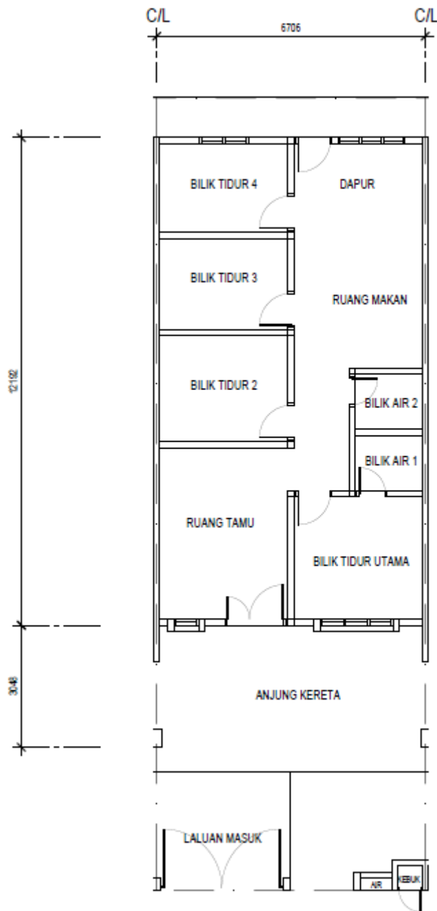
PELAN LANTAI
