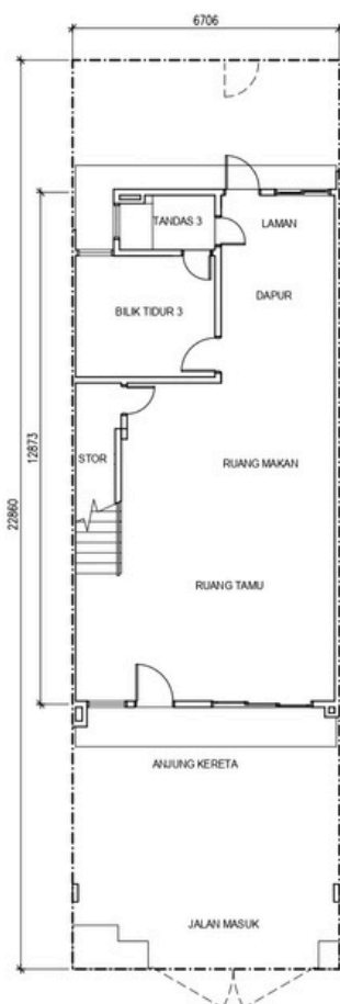
PELAN TINGKAT BAWAH
