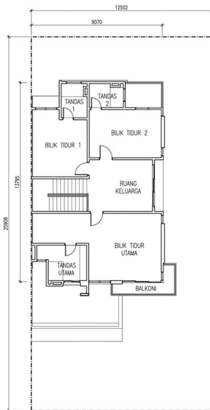
PELAN TINGKAT SATU
