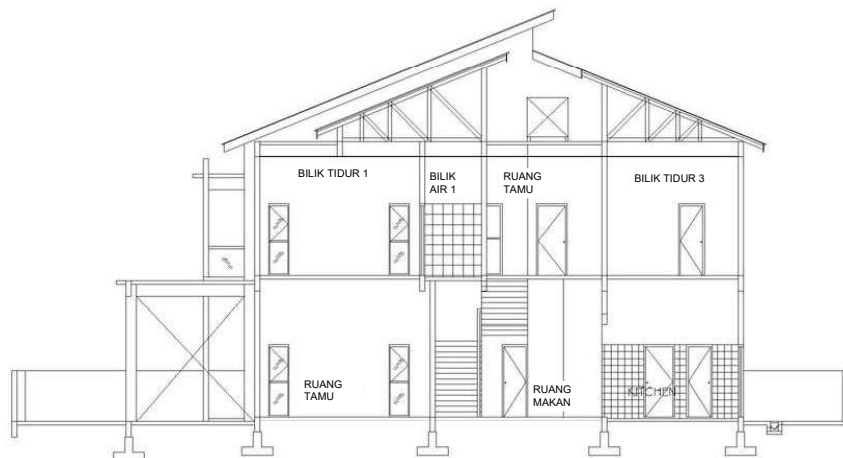
KERATAN A-A
