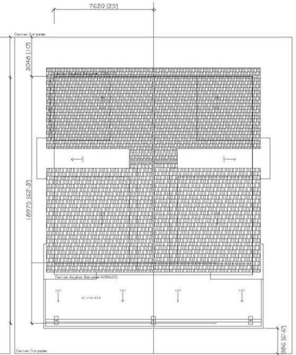
PELAN BUMBUNG
