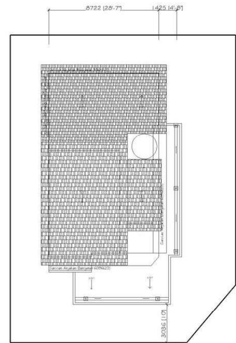
PELAN BUMBUNG
