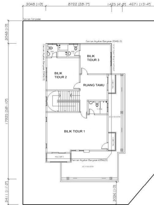
PELAN ARAS 1
