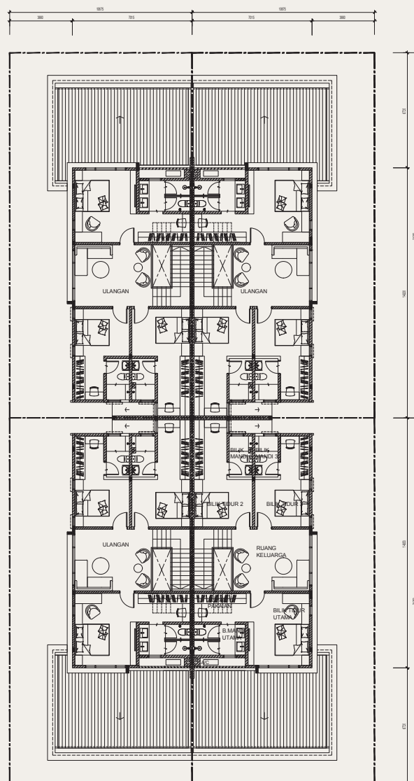
Tingkat Atas
