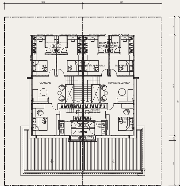
Tingkat Atas
