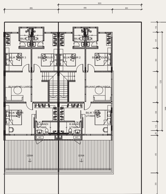
Tingkat Atas
