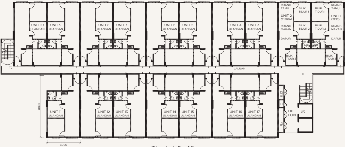
Tingkat 2 - 10
