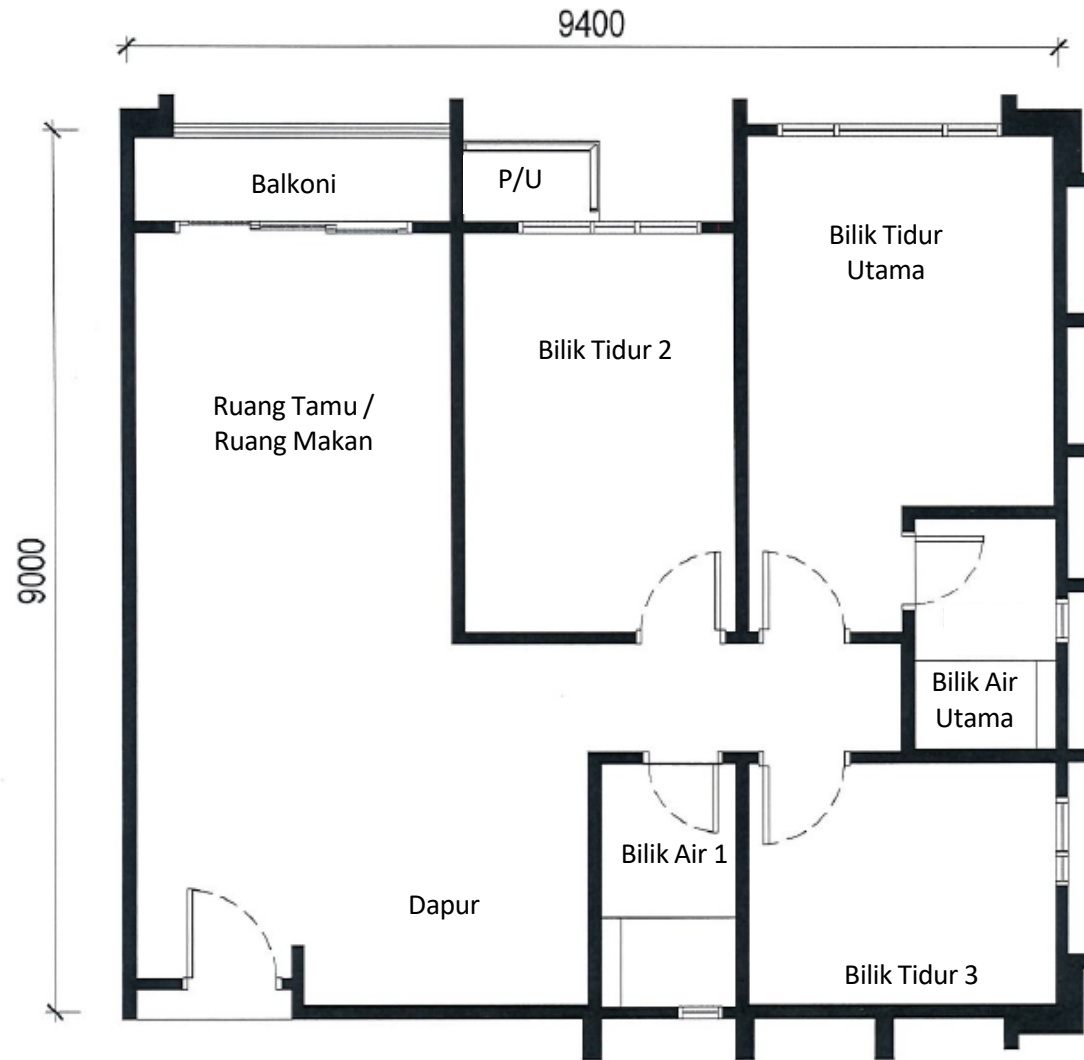
Pelan Lantai Jenis C1a- 82 Meter Persegi (37 Unit)
