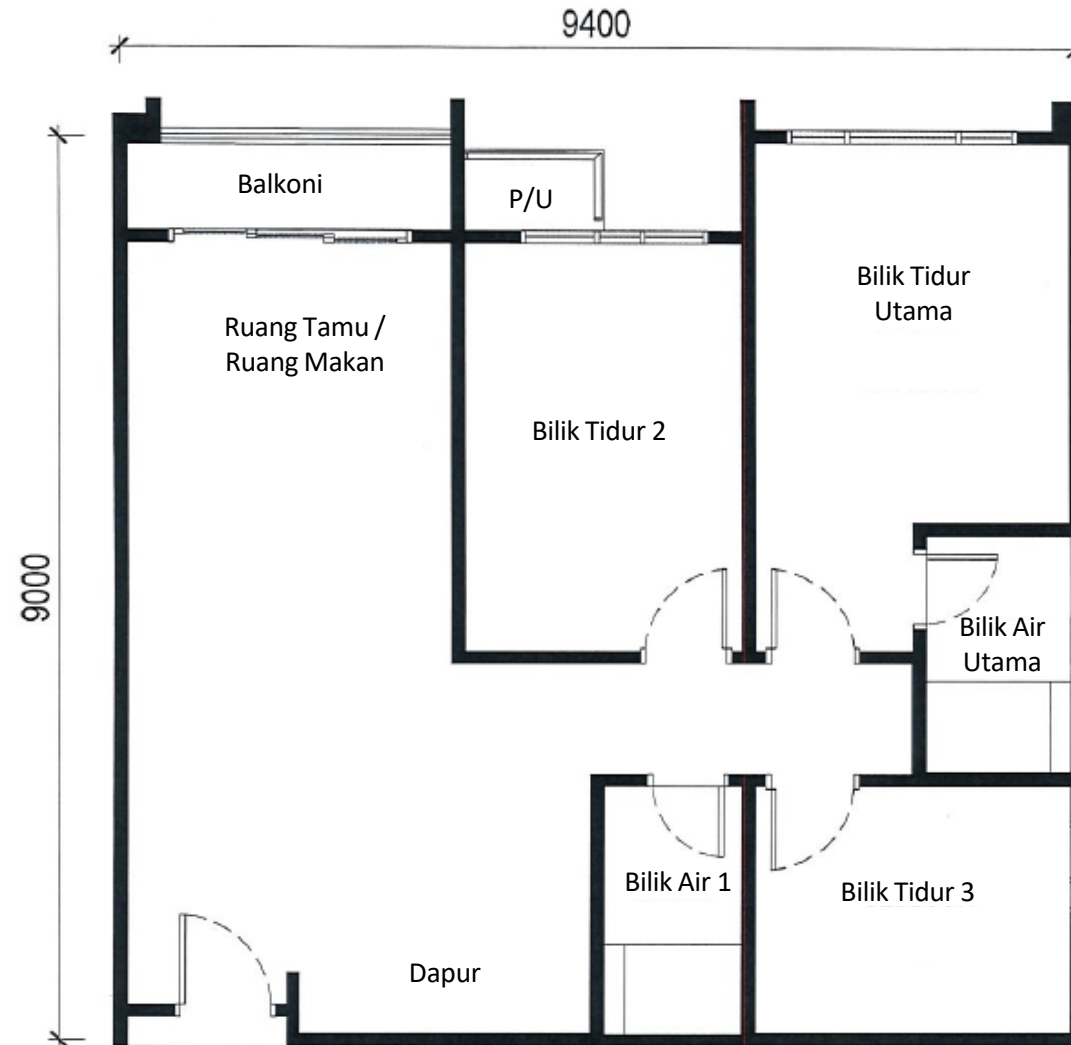
Pelan Lantai Jenis C- 82 Meter Persegi (44 Unit)
