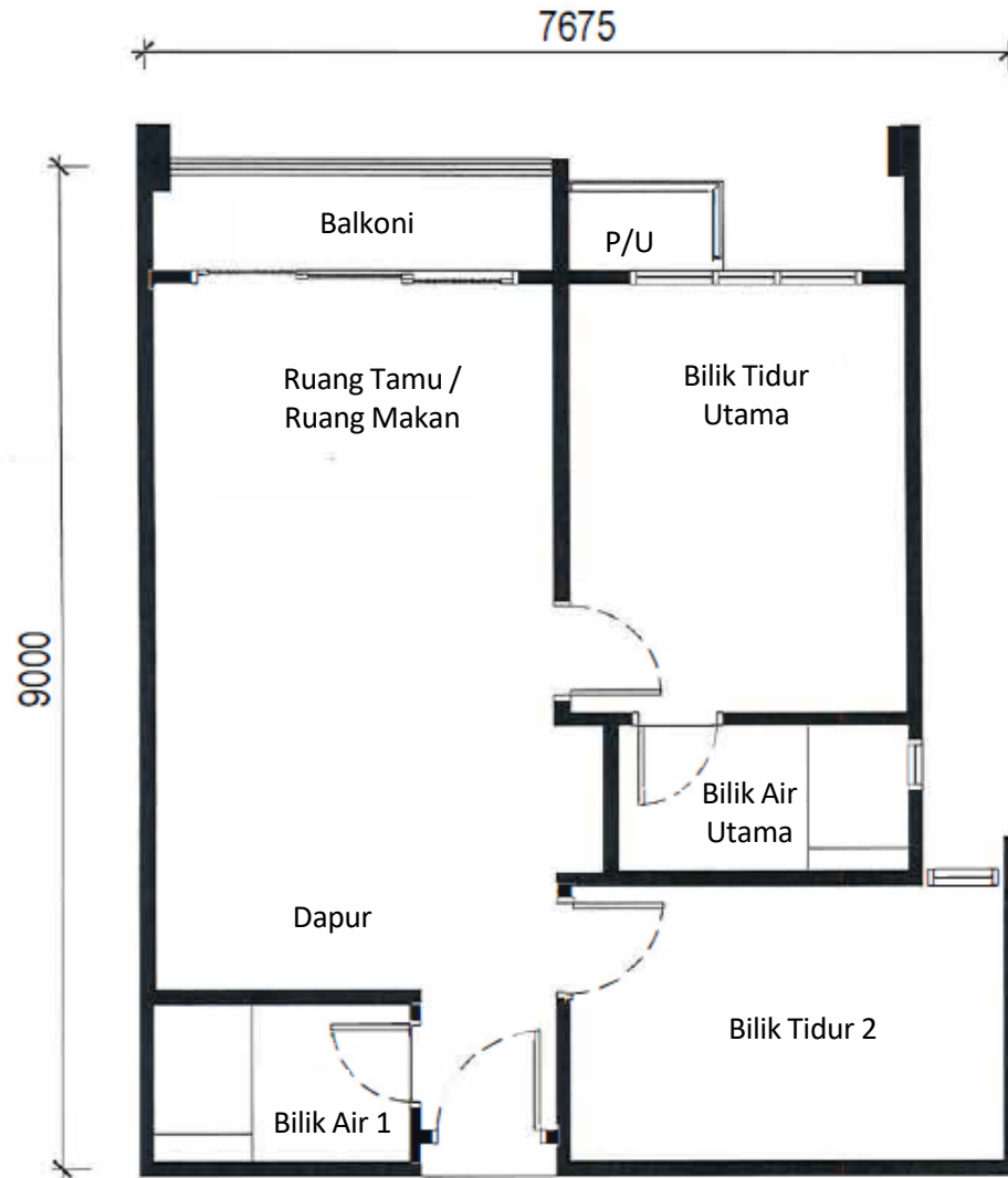
Pelan Lantai Jenis B1-1 – 61 Meter Persegi (81 Unit)
