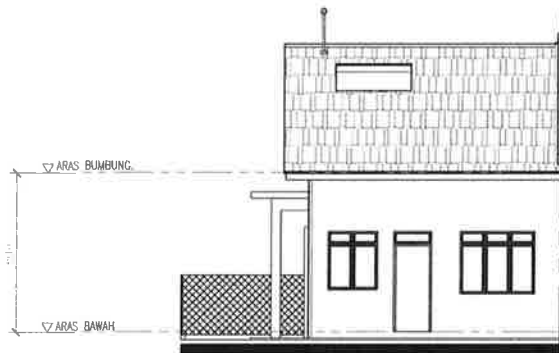
PANDANGAN BELAKANG
