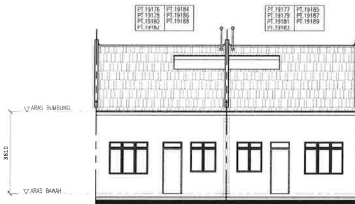
PANDANGAN BELAKANG
