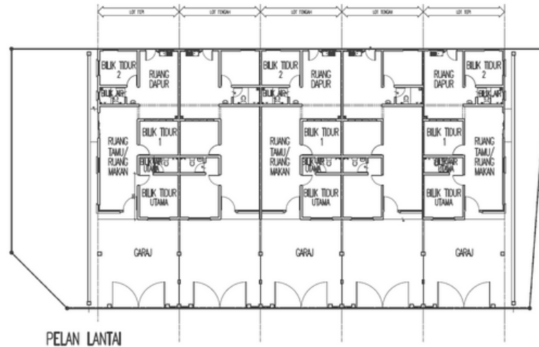
JADUAL KEDUA-PELAN BANGUNAN RUMAH TERES SATU TINGKAT
