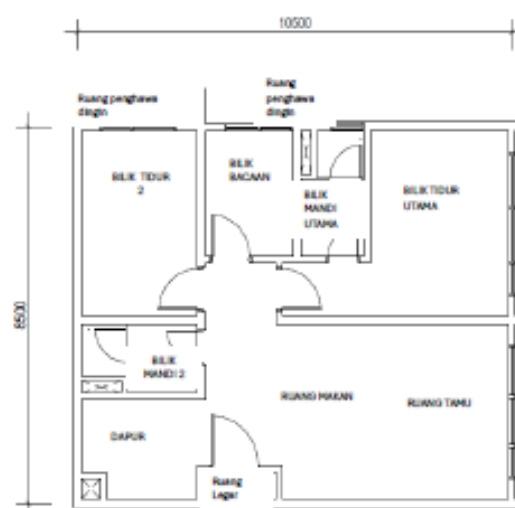
Jenis D3 2 bilik tidur, 1 bilik bacaan, 2 bilik mandi
