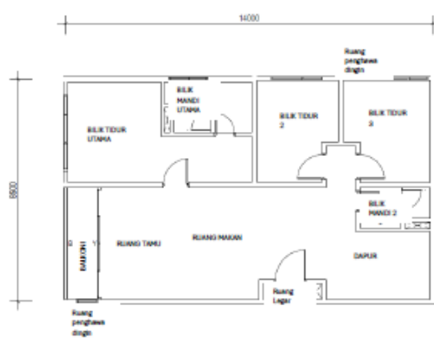
Jenis E2 3 bilik tidur, 2 bilik mandi
