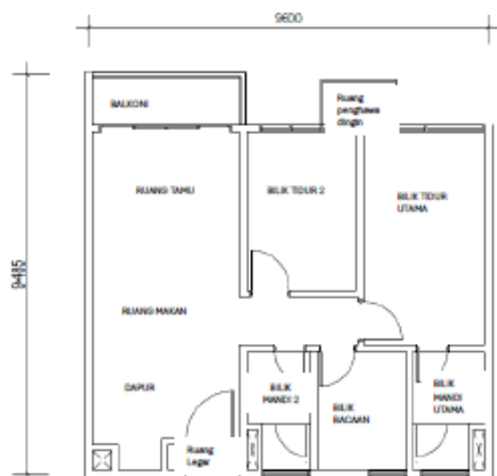
Jenis D2 2 bilik tidur, 1 bilik bacaan, 2 bilik mandi
