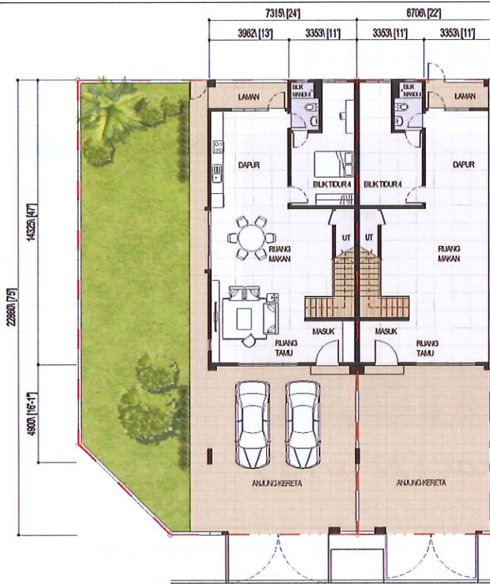
Pelan Lantai Tipikal Tingkat Bawah
