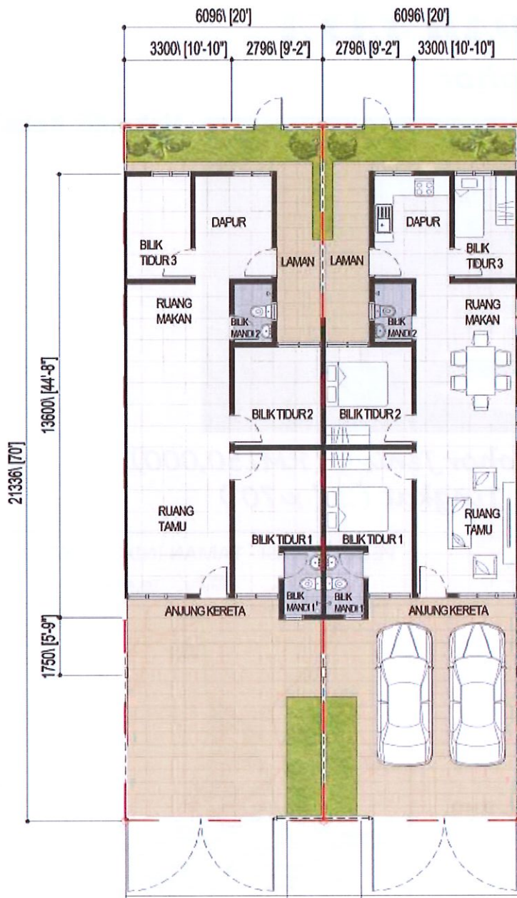
Pelan Lantai Tipikal
