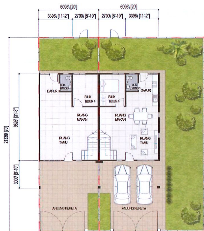
Pelan Lantai Tipikal Tingkat Bawah
