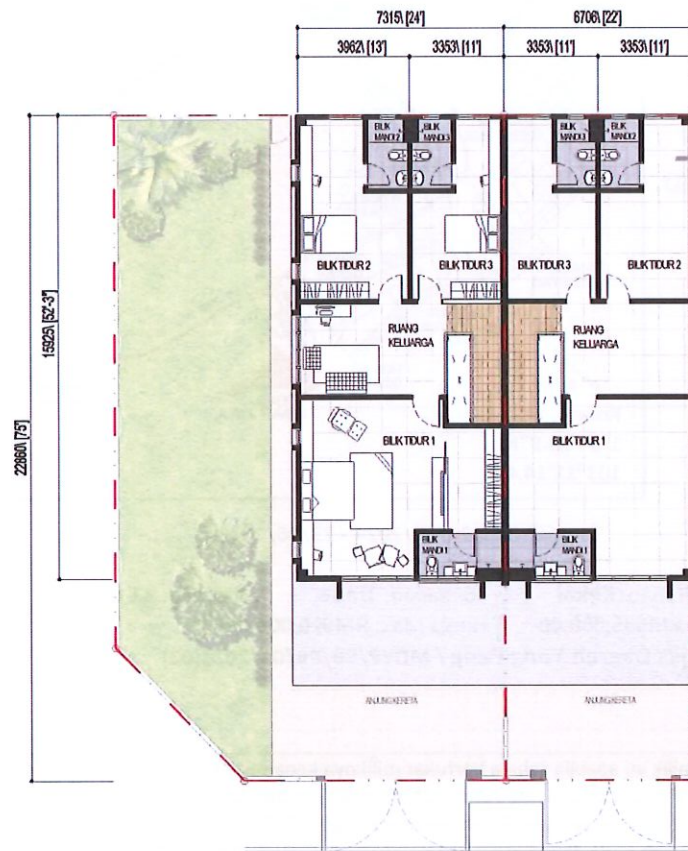
Pelan Lantai Tipikal Tingkat Atas
