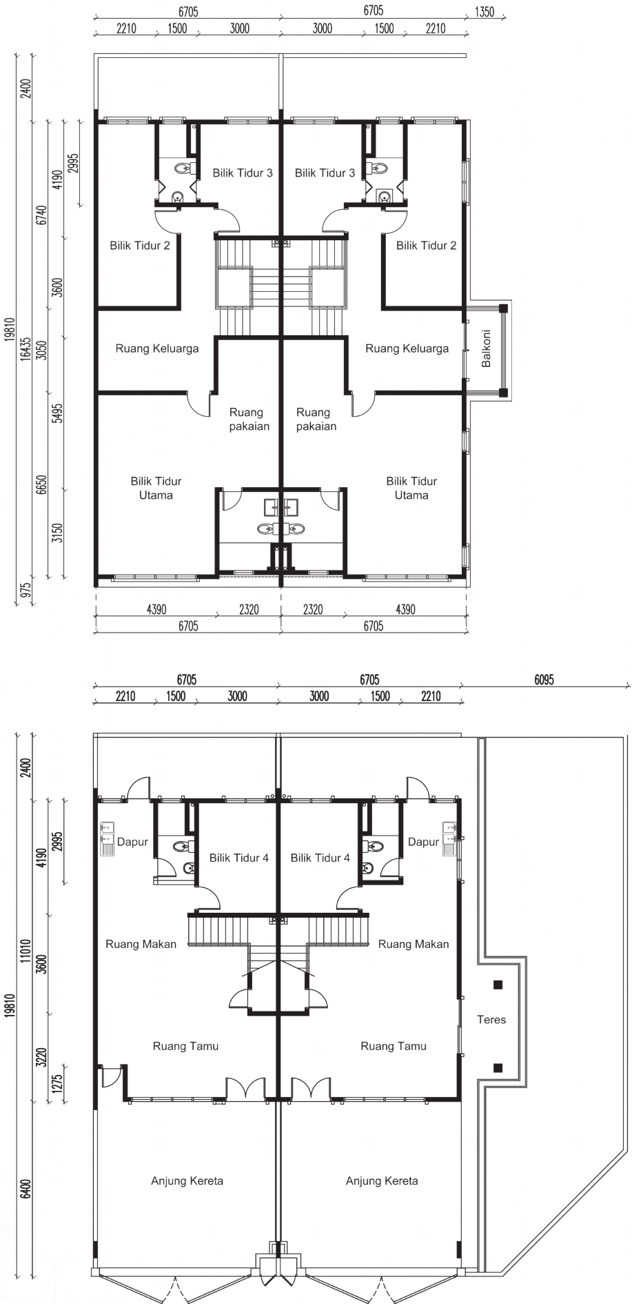
PELAN LANTAI
