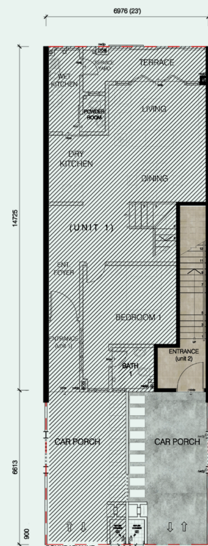
PELAN TINGKAT BAWAH SKALA 1:100
