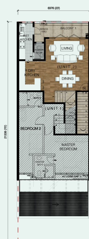
PELAN TINGKAT SATU SKALA 1:100
