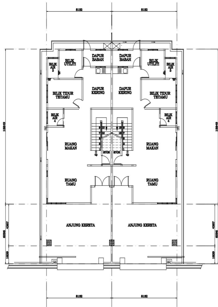
1. PELAN LANTAI TINGKAT BAWAH RUMAH BERKEMBAR 2 TINGKAT
