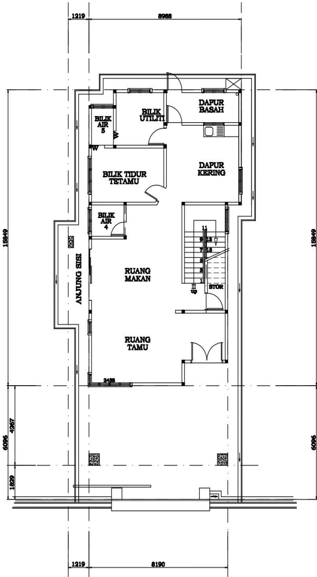
1. PELAN LANTAI TINGKAT BAWAH RUMAH BANGLO 2 TINGKAT
