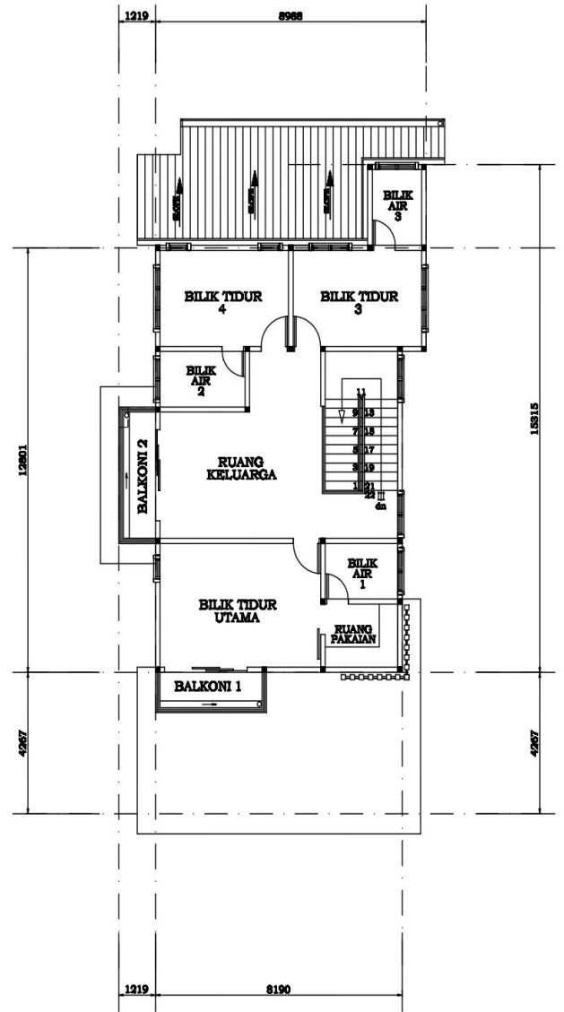
2. PELAN LANTAI TINGKAT ATAS
