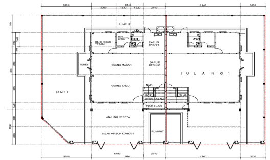
PELAN LANTAI TINGKAT BAWAH
