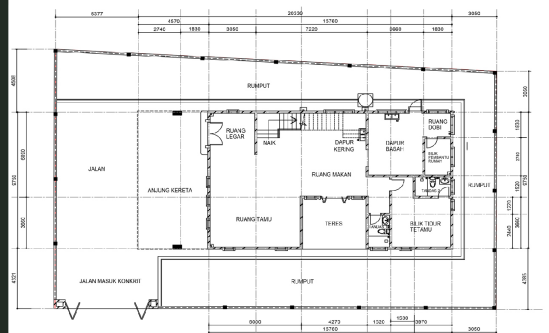
PELAN LANTAI TINGKAT BAWAH Rumah Banglo 2 Tingkat
