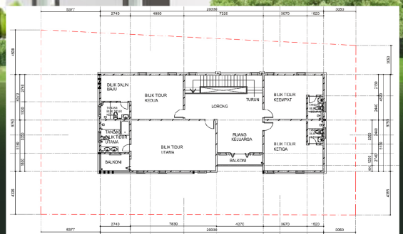
PELAN LANTAI TINGKAT SATU Rumah Banglo 2 Tingkat
