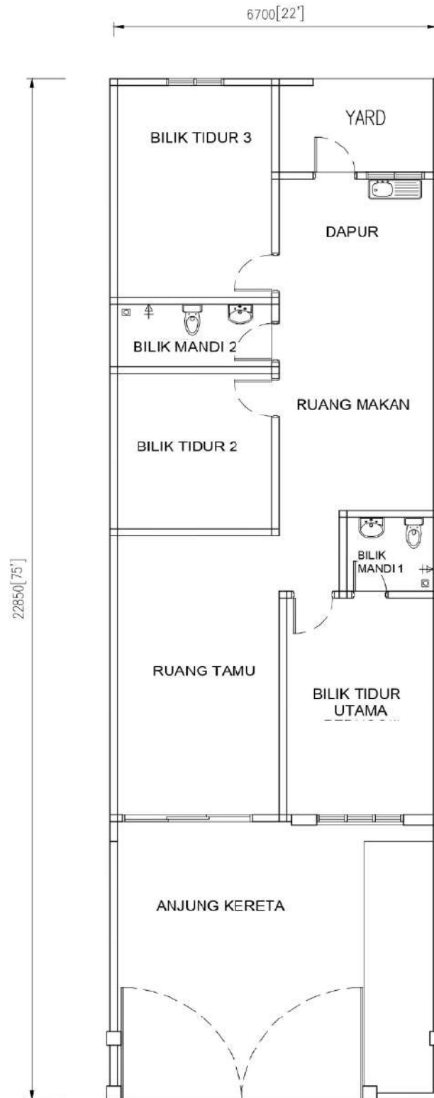
PELAN LANTAI TINGKAT BAWAH RUMAH TERES SATU TINGKAT JENIS D - 22'X75'
