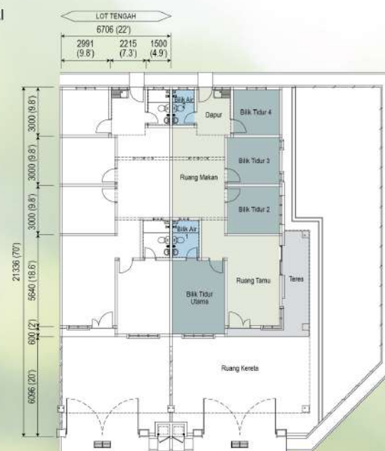
PELAN LANTAI
