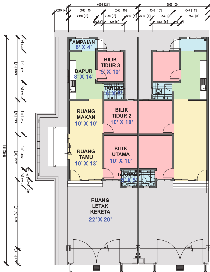
PELAN LANTAI: DARI 1195 KAKI PERSEGI
