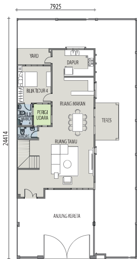
PELAN TINGKAT BAWAH
