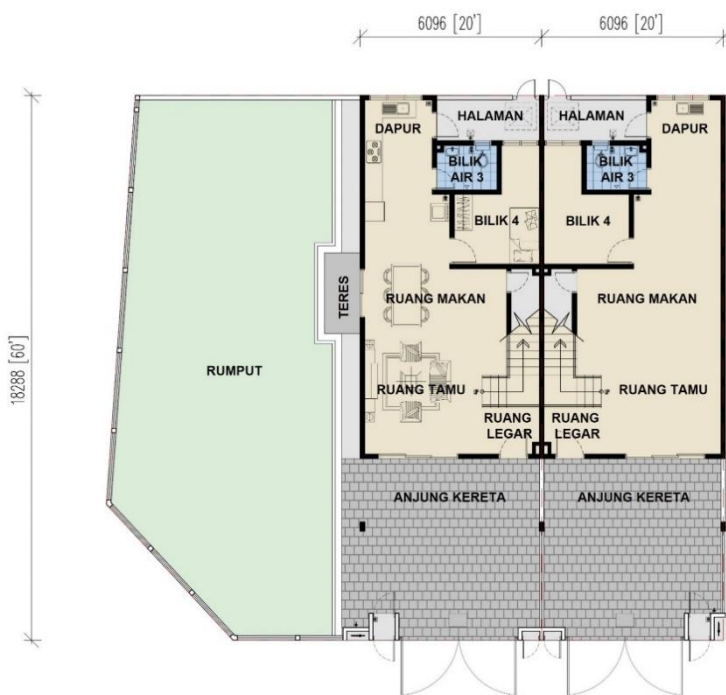
PELAN LANTAI BAWAH (20' X 60')
