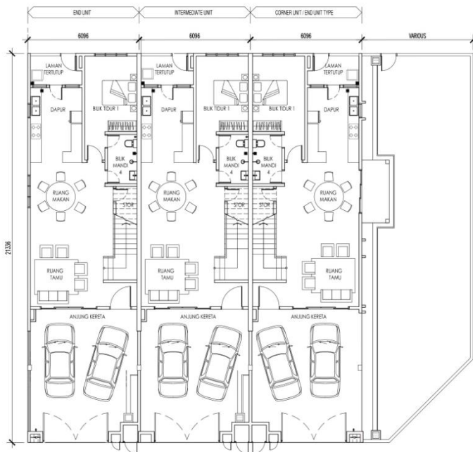
Tingkat Bawah
