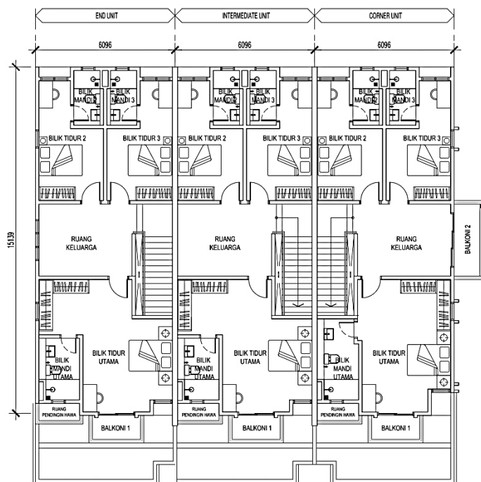
Tingkat Satu
