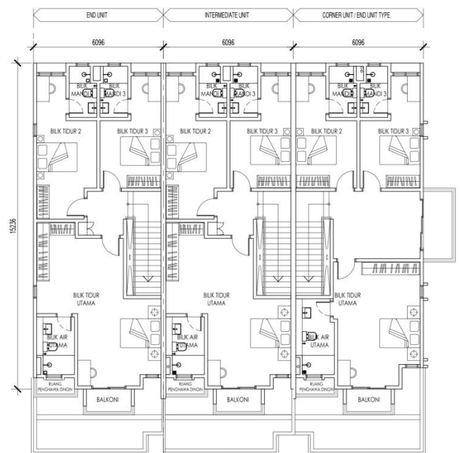
Tingkat Satu
