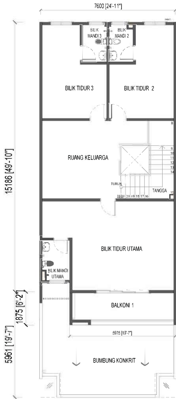
ARAS LANTAI TINGKAT SATU
