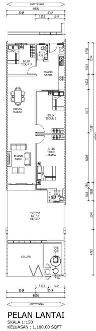
TERES 1 TINGKAT - UNIT TENGAH
