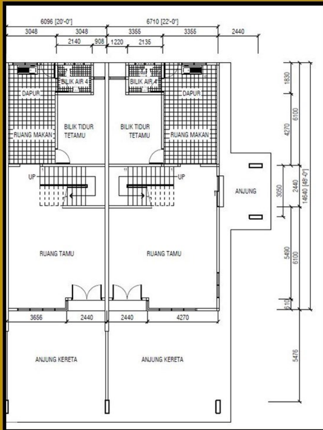
TINGKAT BAWAH
