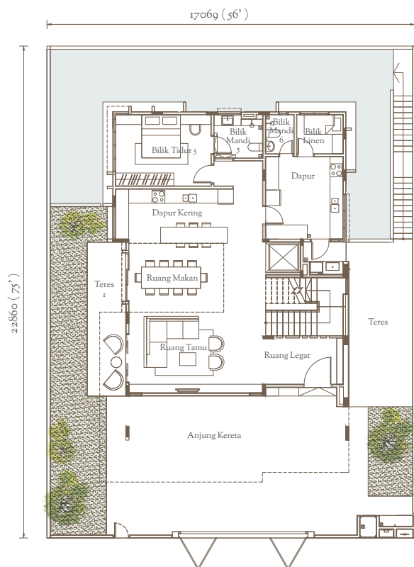
Tingkat Bawah
