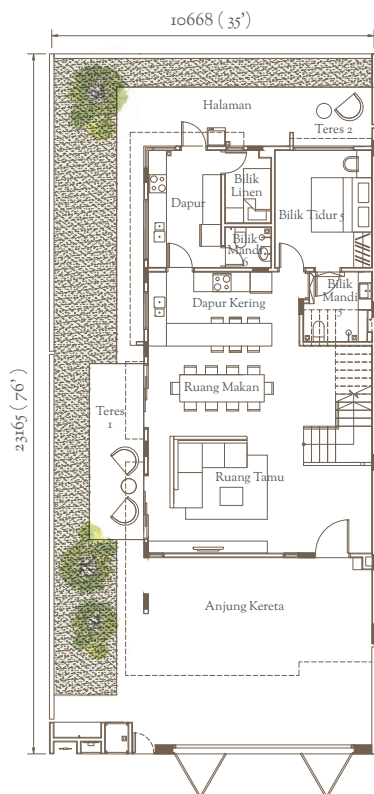
Tingkat Bawah
