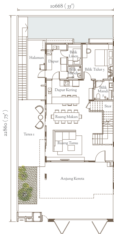
Tingkat Bawah
