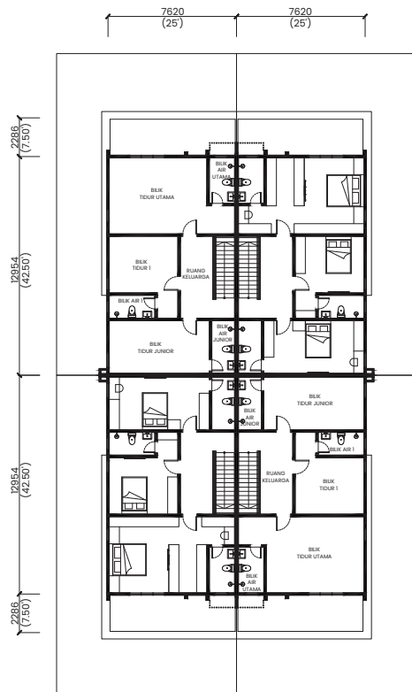
TINGKAT SATU
