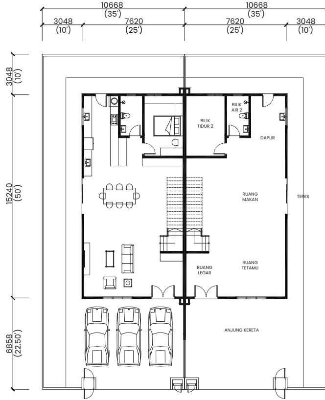
TINGKAT BAWAH
