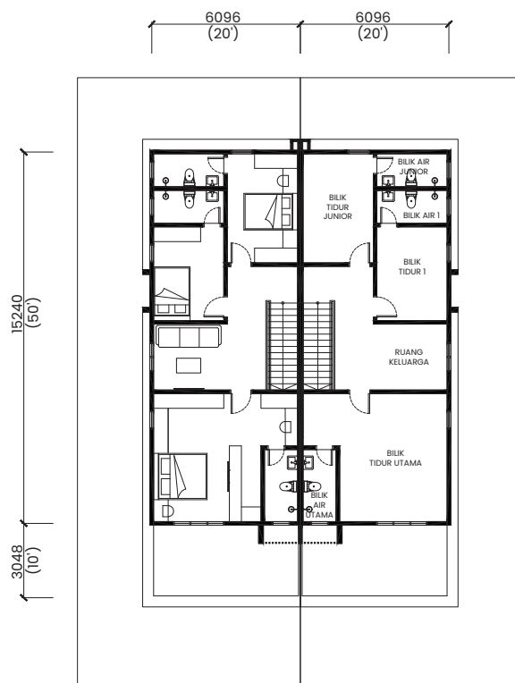
TINGKAT SATU
