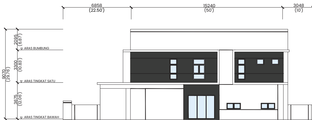
PANDANGAN SISI
