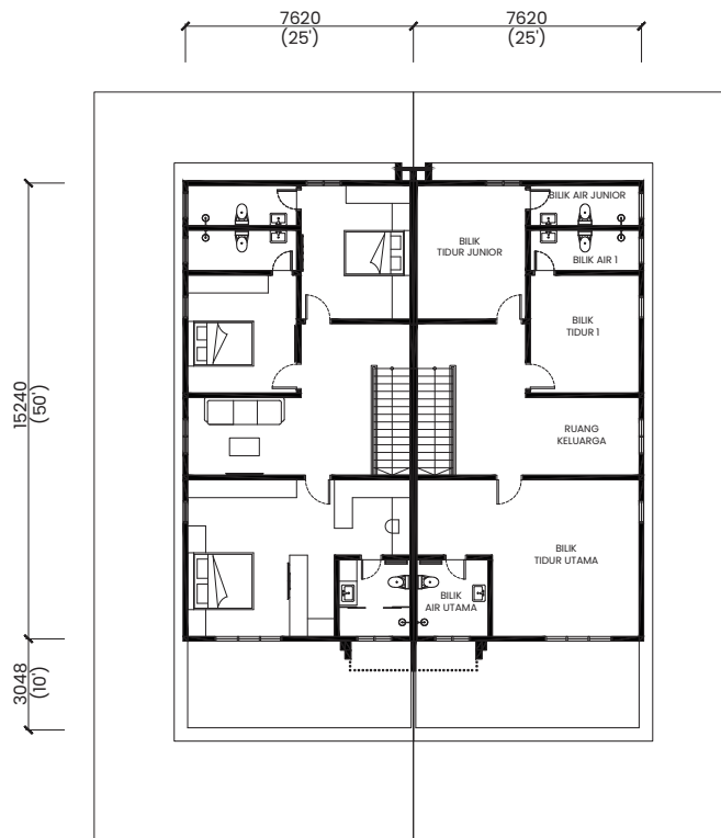
TINGKAT SATU
