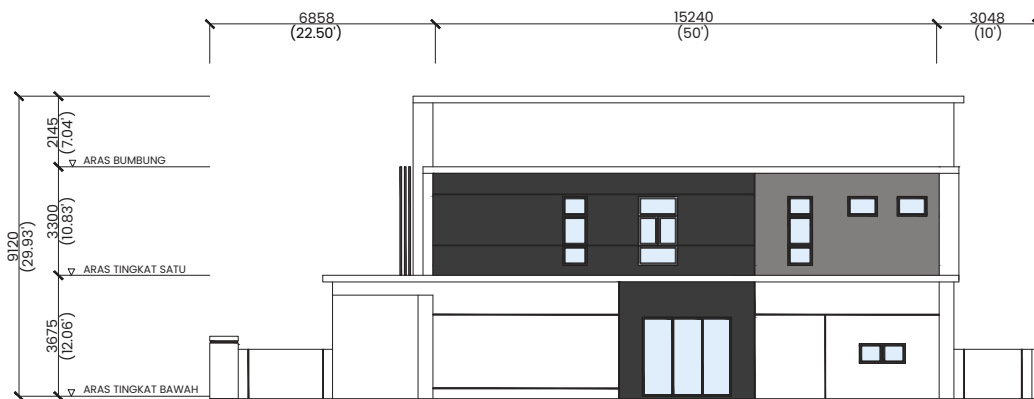
PANDANGAN SISI
