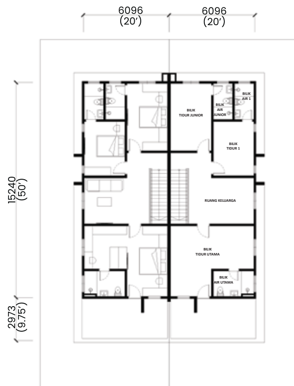
TINGKAT SATU
