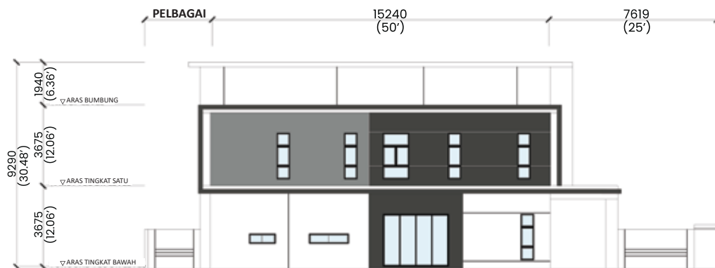
PANDANGAN SISI
