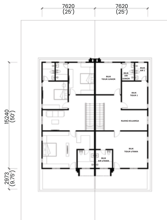
TINGKAT SATU
