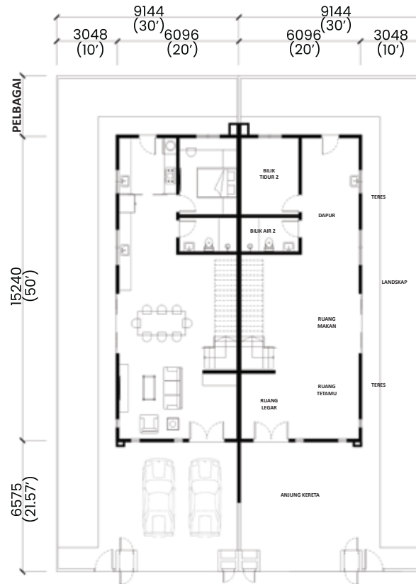
TINGKAT BAWAH
