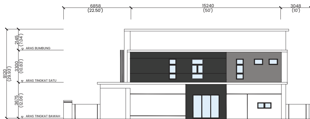
PANDANGAN SISI
