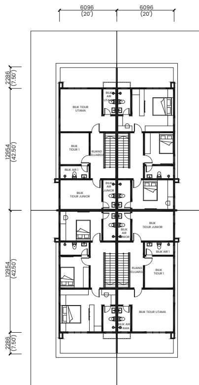
TINGKAT SATU
