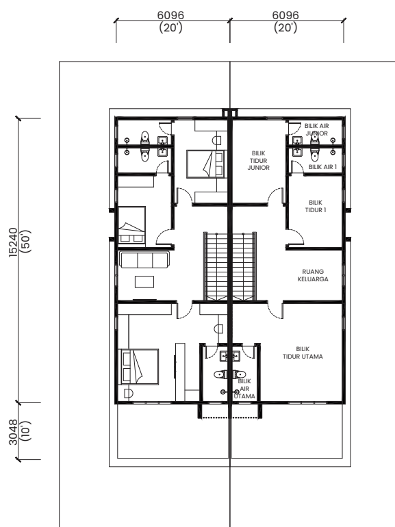
TINGKAT SATU
