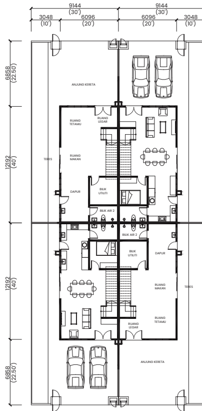
TINGKAT BAWAH
