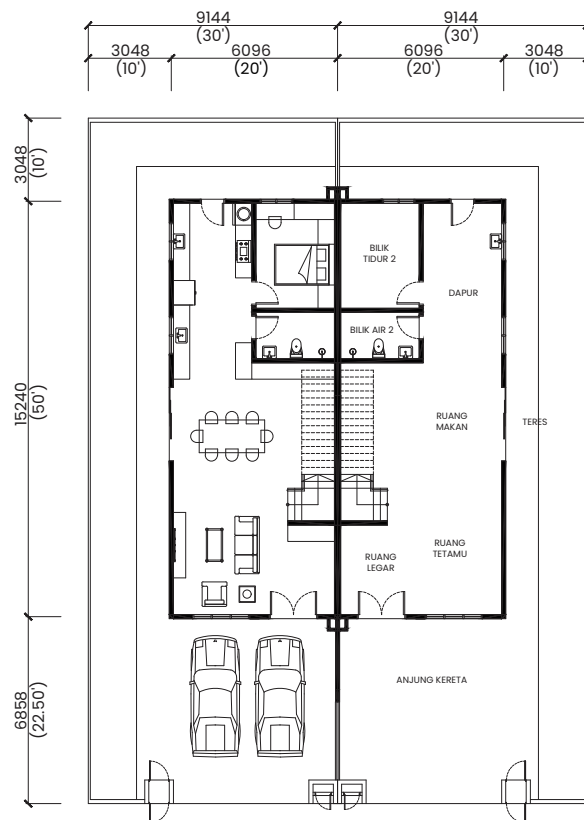
TINGKAT BAWAH
