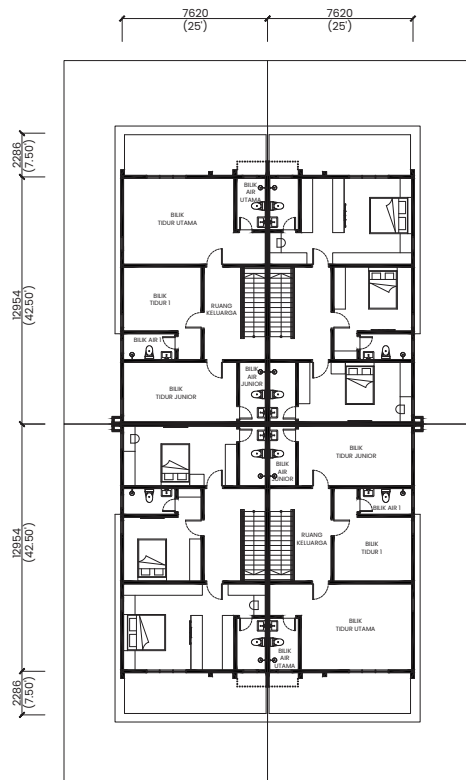
TINGKAT SATU
