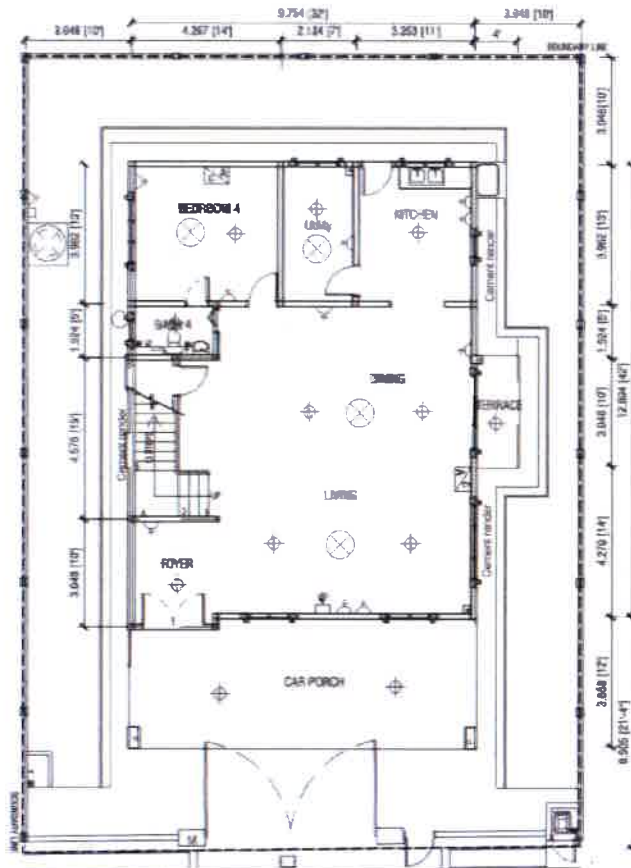
TINGKAT BAWAH PTD. 27836-PTD 27840
