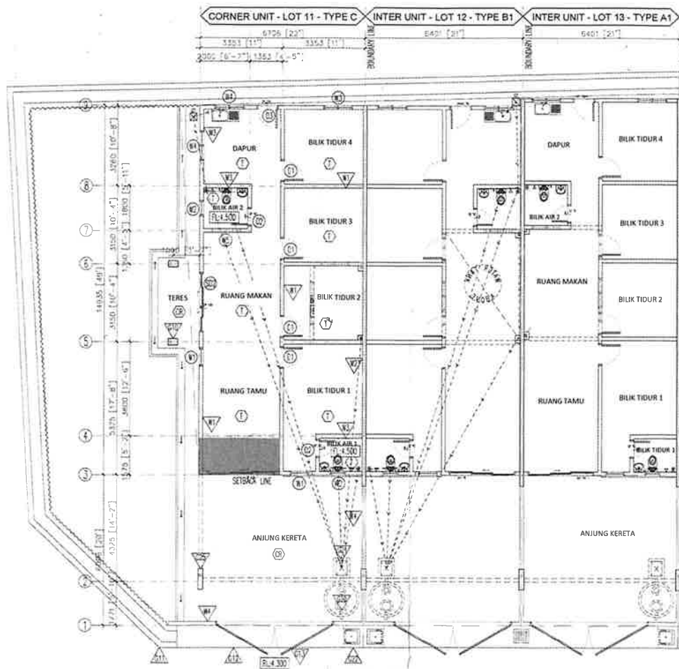
PELAN LANTAI
