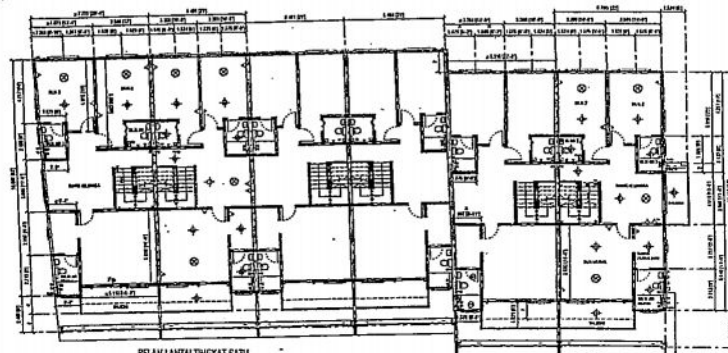
PELAN LANTAI TINGKAT SATU RUMAH TERES
