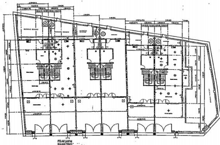
PELAN LANTAI RUMAH TERES
