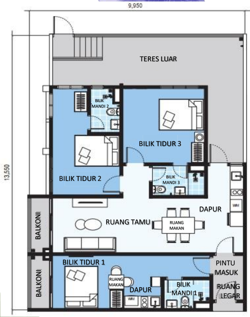
JENIS D1 1,370 KAKI PERSEGI
