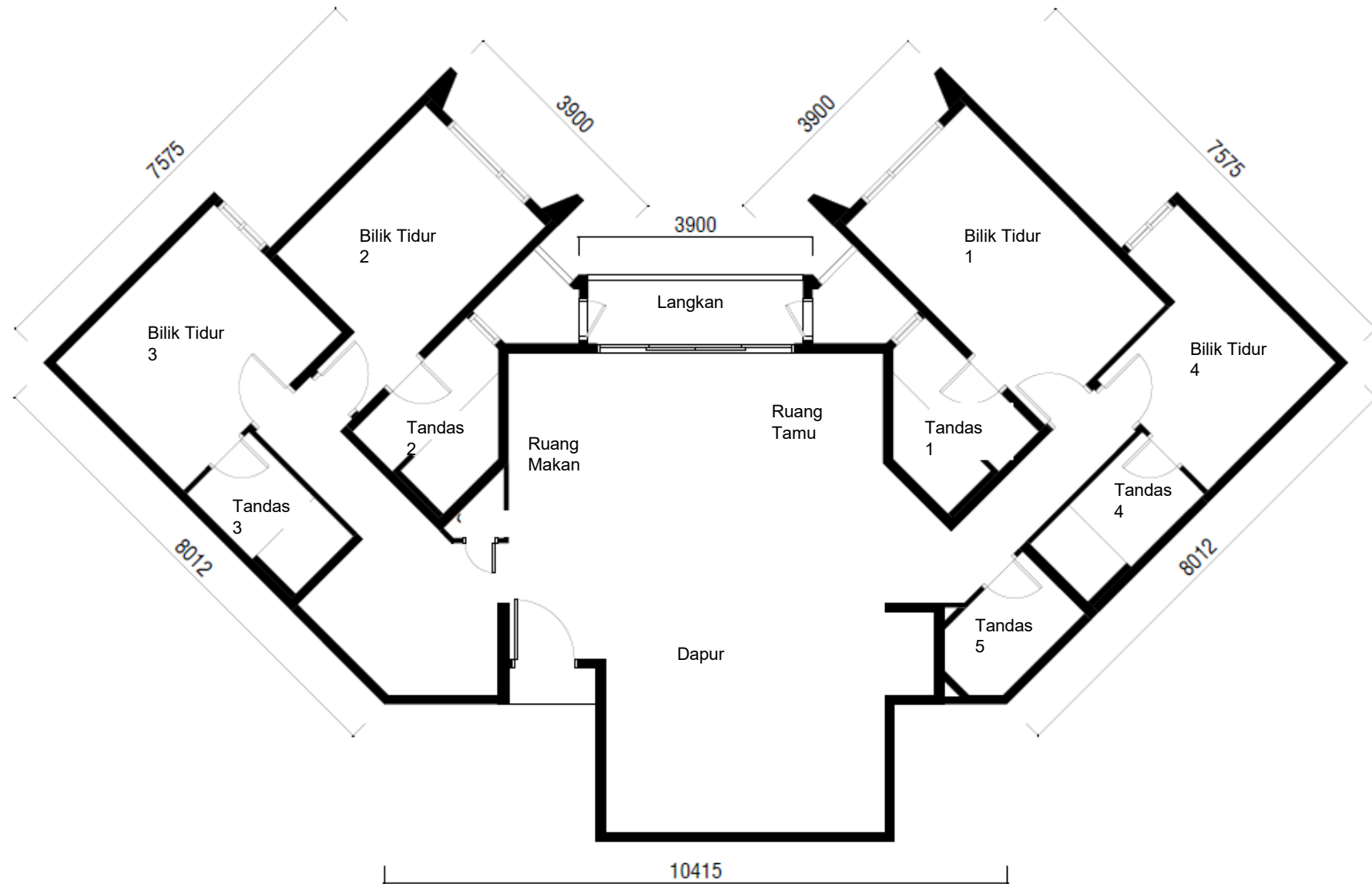
Pelan Lantai Jenis C – 150 meter persegi (37 unit)
