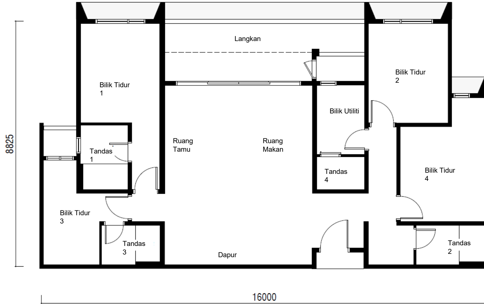
Pelan Lantai Jenis B2-1 – 132 meter persegi (9 unit)
