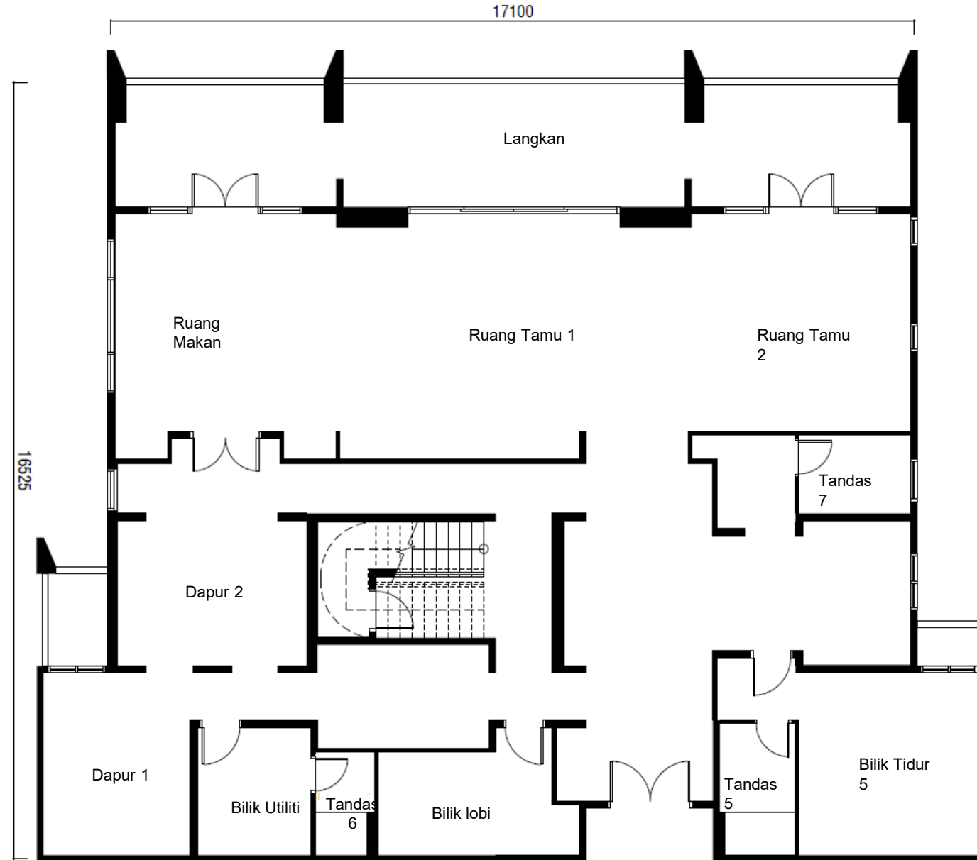
Pelan Lantai Jenis F - Tingkat bawah – 299 meter persegi (37 unit)
