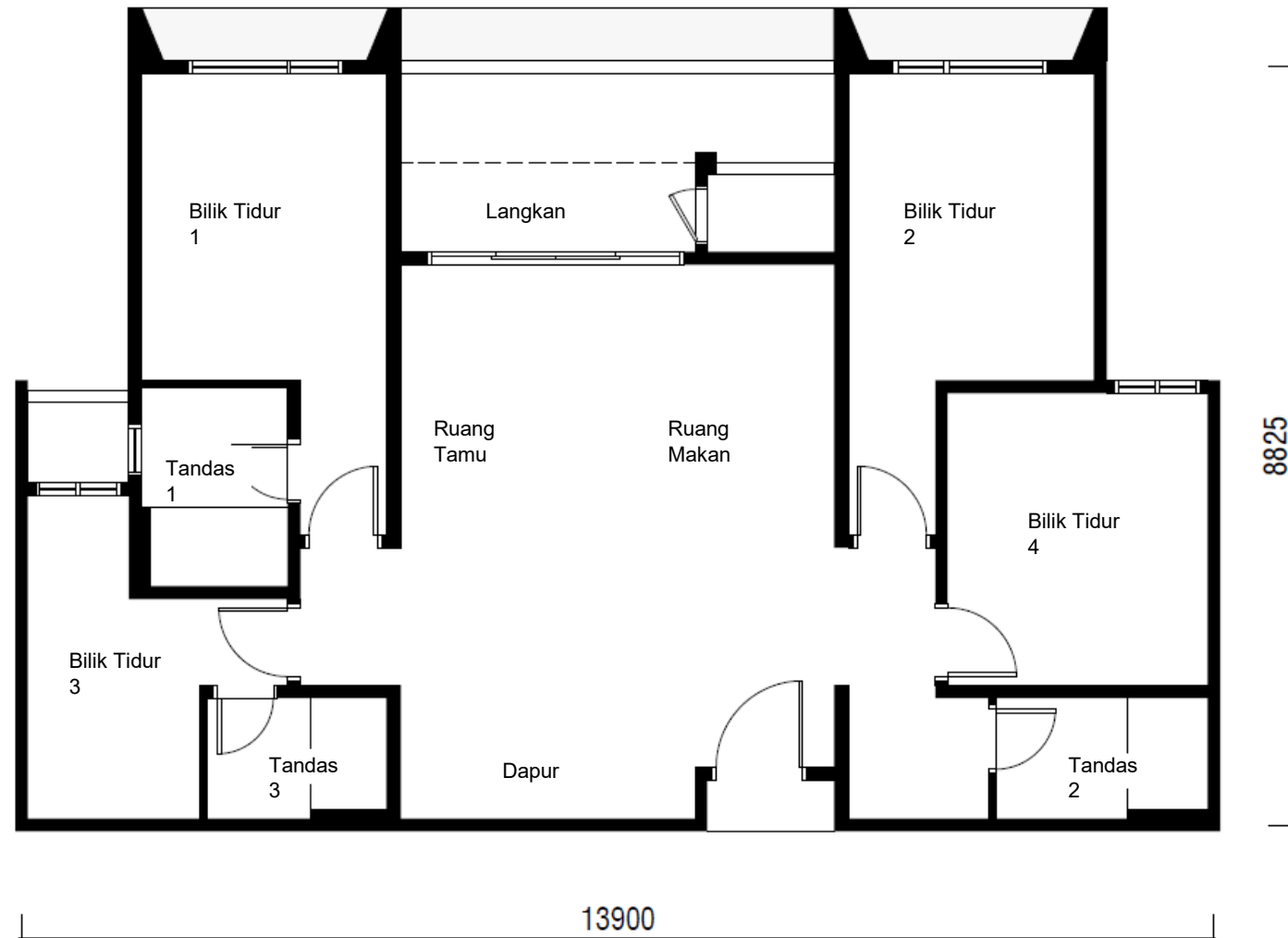
Pelan Lantai Jenis A-1 - 112 meter persegi (47 unit)
