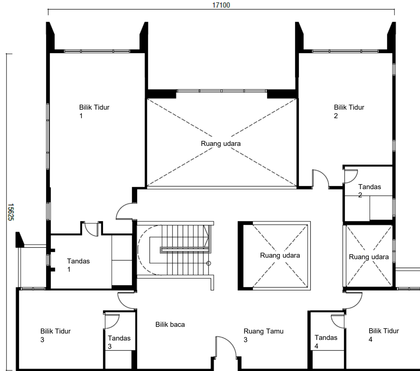
Pelan Lantai Jenis F - Tingkat atas – 214 meter persegi
