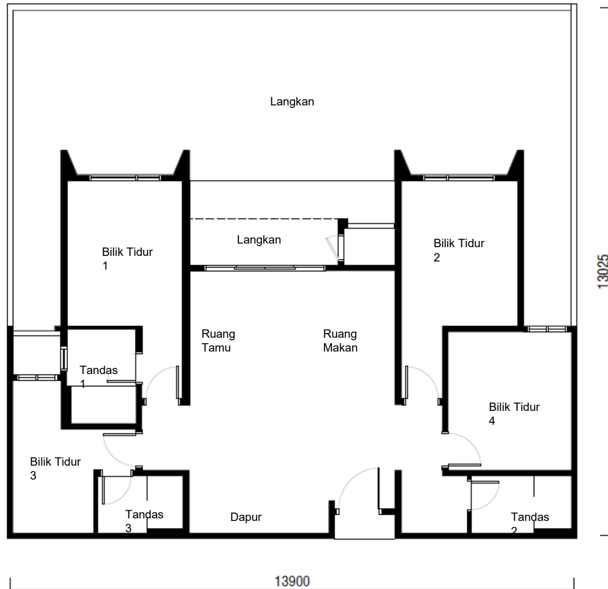
Pelan Lantai Jenis A3 - 180 meter persegi (1 unit)
