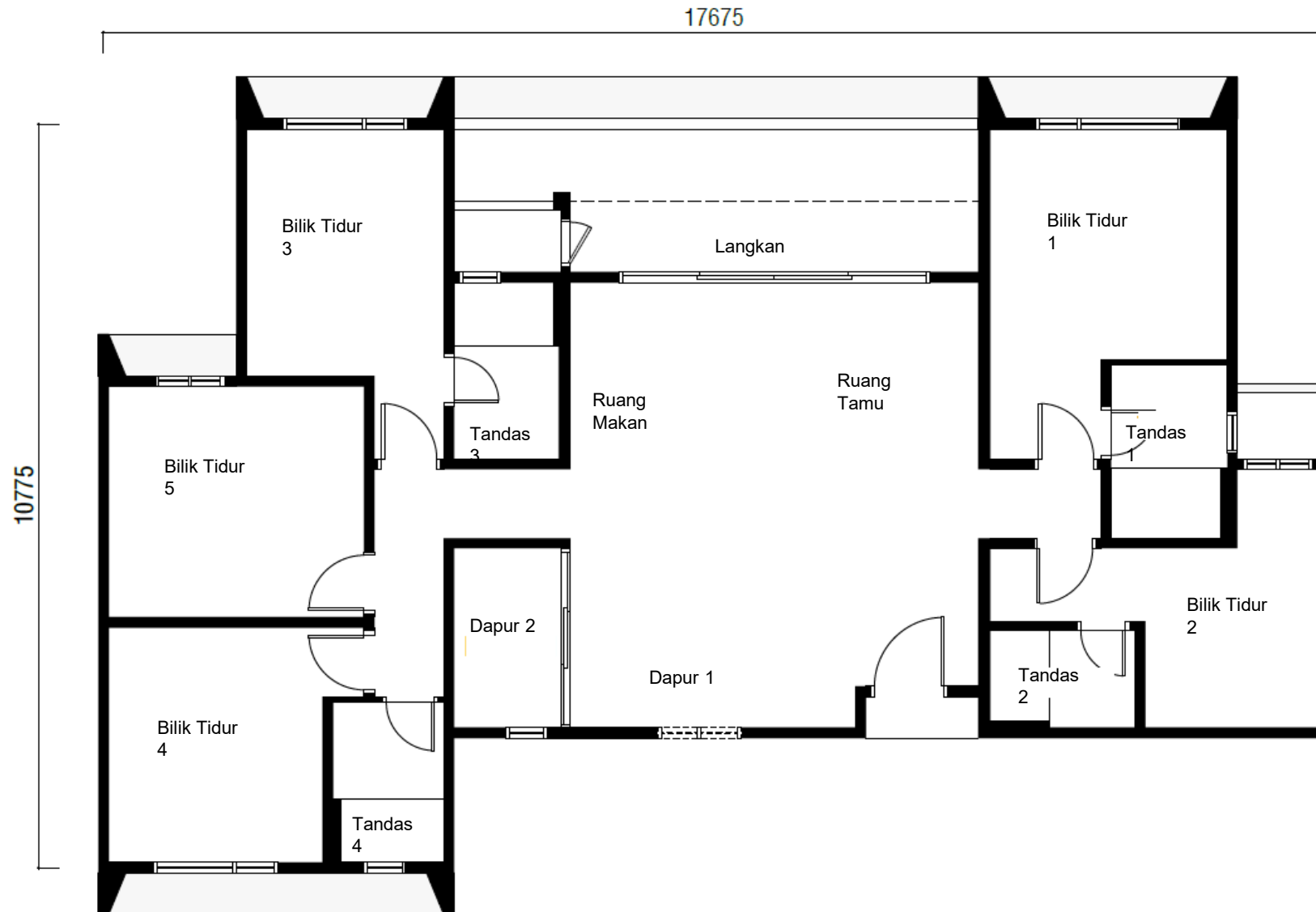
Pelan Lantai Jenis D-1 – 153 meter persegi (20 unit)
