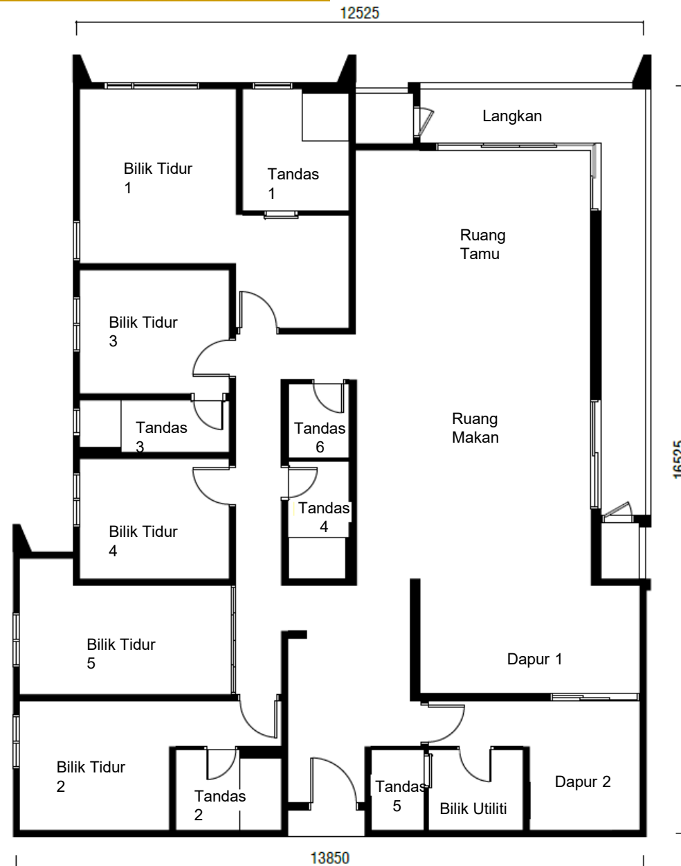
Pelan Lantai Jenis E – 216 meter persegi (38 unit)
