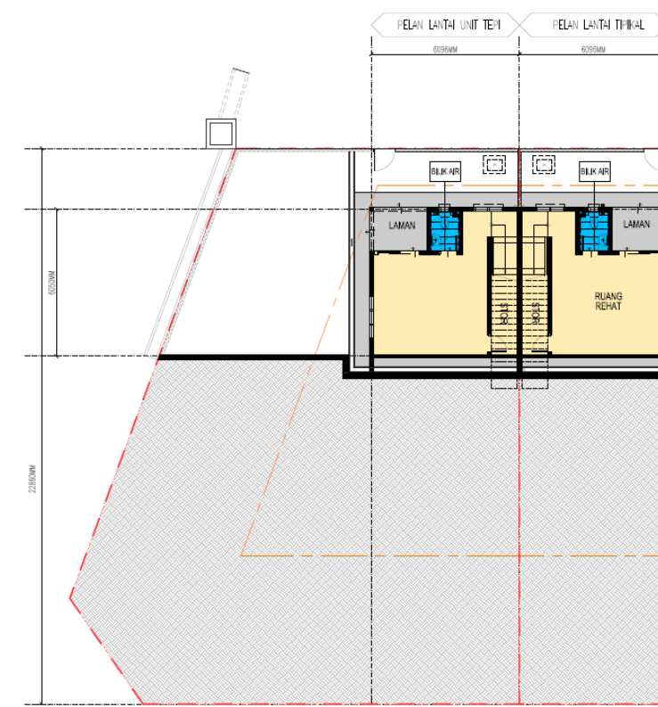
Tingkat Bawah
