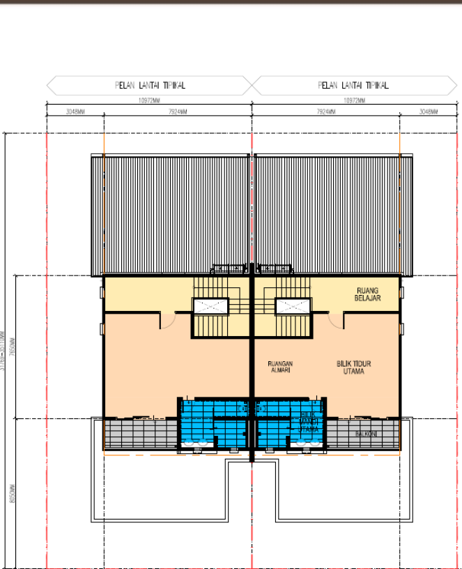
Tingkat Dua
