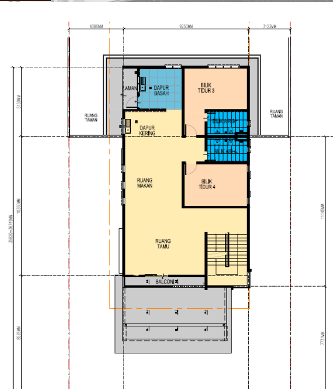
Tingkat Satu
